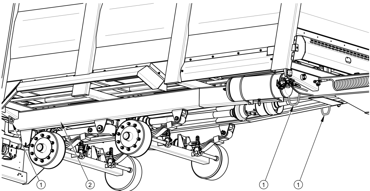
RYСУNEK 1.3 Rozmieszczenie uchwytów transportowych
