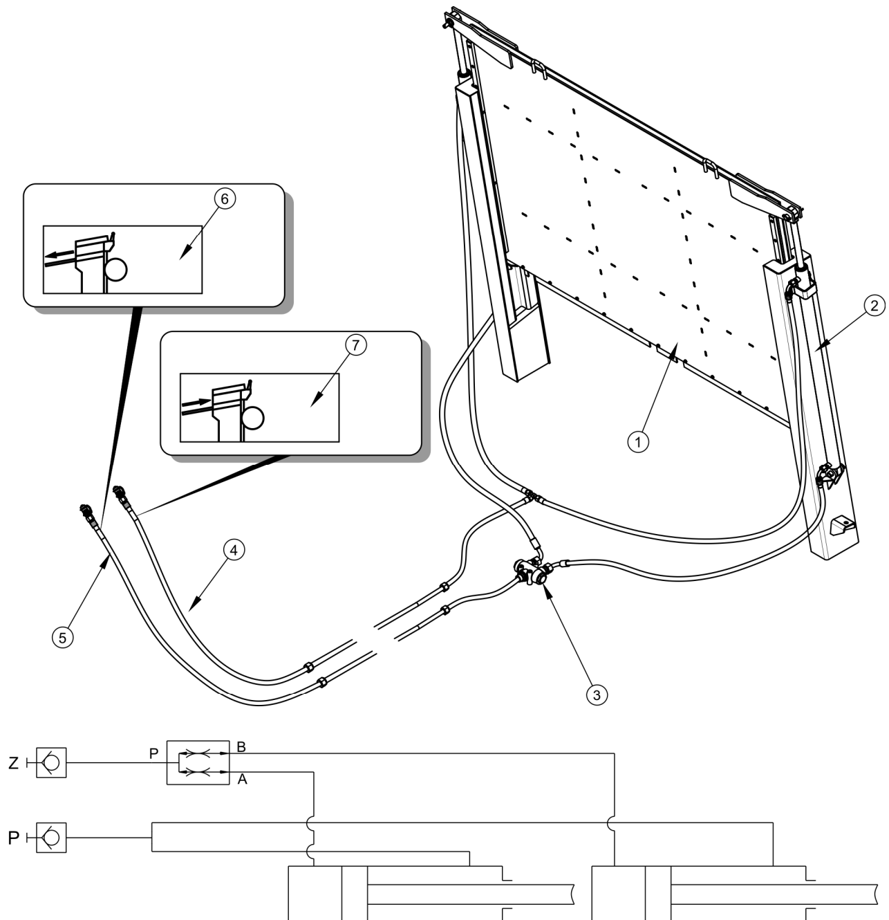
RYСУNEK 3.6 Budowa i schemat instalacji hydraulicznej zasuwy
