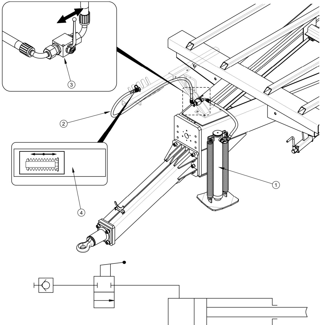
RYСУNEK 3.4 Budowa i schemat instalacji hydraulicznej podpory prostej
