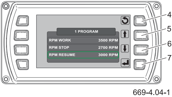
Rysunek 4.4 Ekran ustawień programów (4) przycisk wyjścia (5) przycisk góra (6) przycisk dół (7) przycisk zatwierdź
