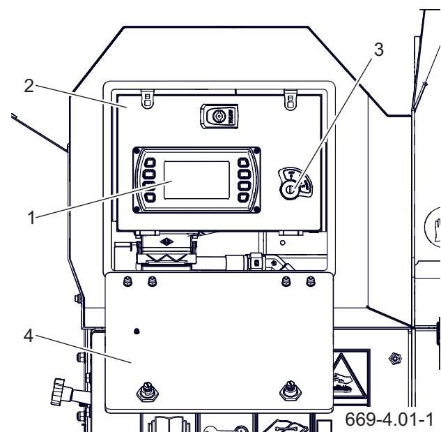
Rysunek 4.1 Położenie panelu sterującego. (1) panel sterujący (2) skrzynka sterownicza (3) stacyjka (4) pokrywa
