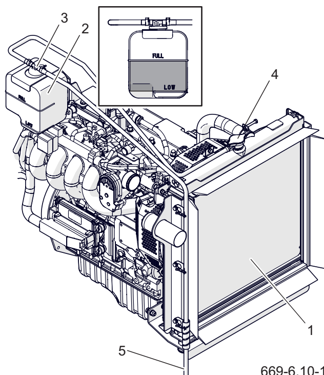
Rysunek 6.6 Układ chłodzenia
