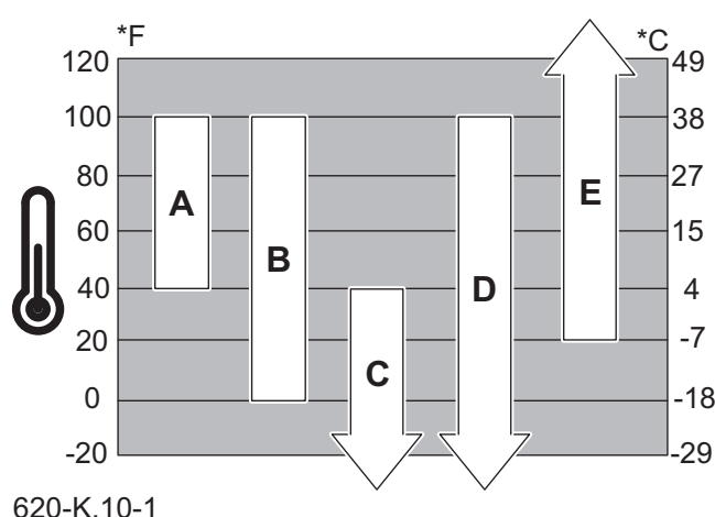
Rysunek 7.10 Klasa lepkości oleju w zależności od temperatury
