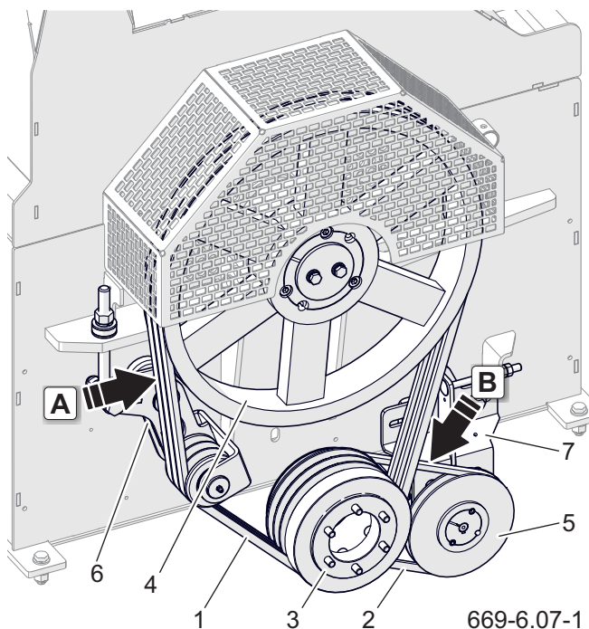
Rysunek 6.20 Pasy napędowe
