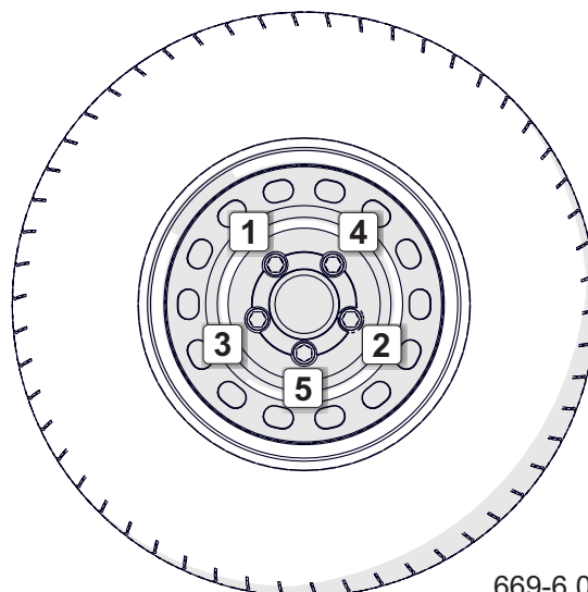
Rysunek 6.19 Kolejność dokręcania śrub
