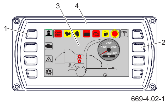
Rysunek 4.2 Budowa panelu sterującego. (1) lewe przyciski nawigacyjne (2) prawe przyciski nawigacyjne (3) wyświetlacz (4) obudowa
