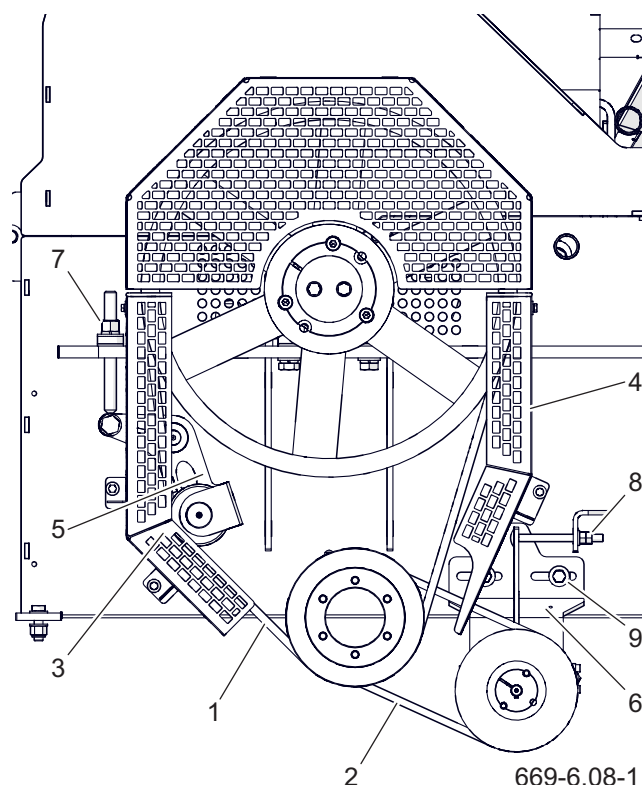
Rysunek 6.21 Przekładnie pasowe
