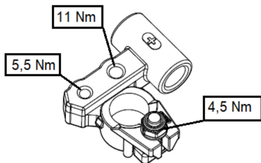
Rysunek 6.12 Klema akumulatora
