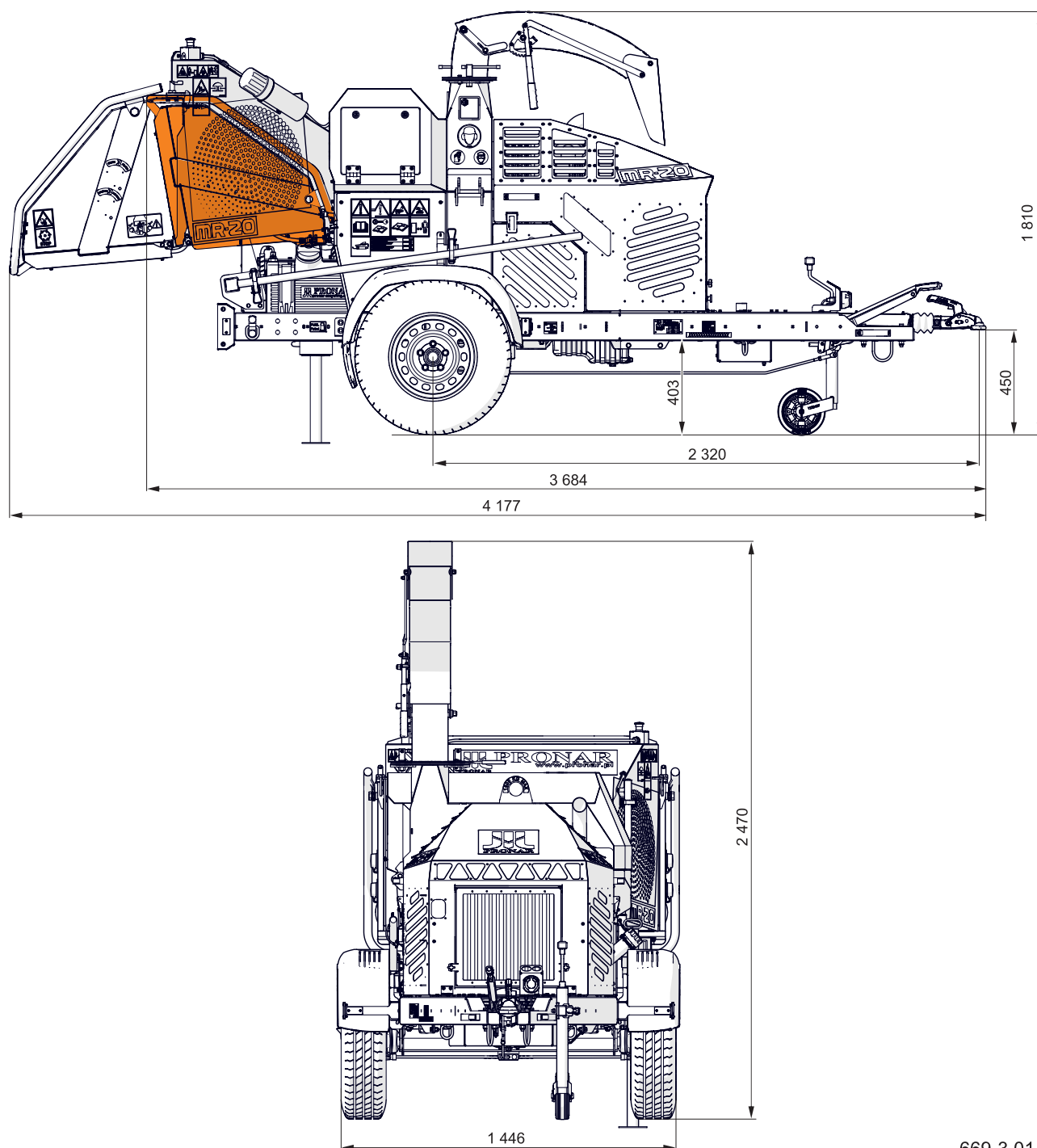
Rysunek 3.1 Wymiary rębaka mobilnego Pronar MR-20
