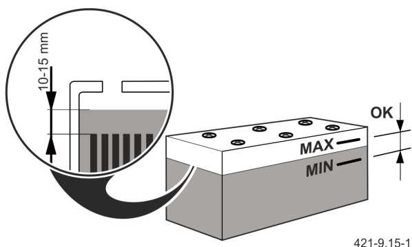
Rysunek 6.11 Kontrola poziomu elektrolitu
