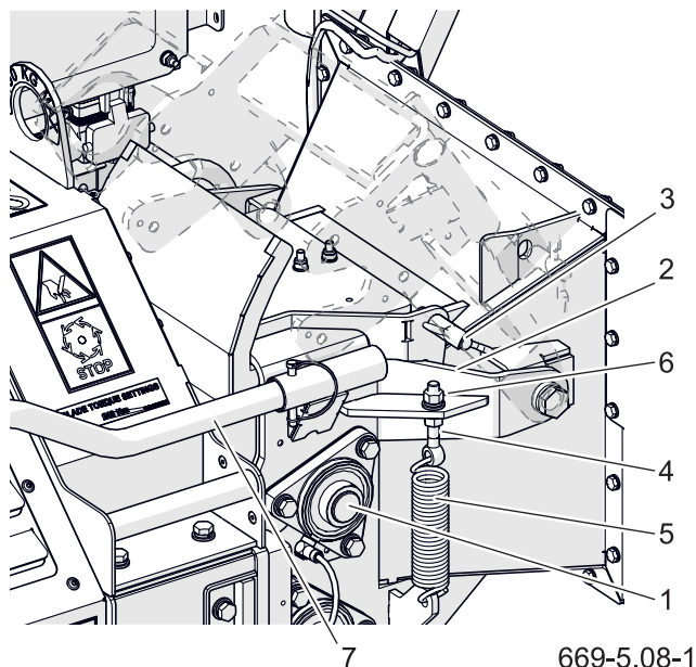
Rysunek 5.10 Rolka górna podnoszona
