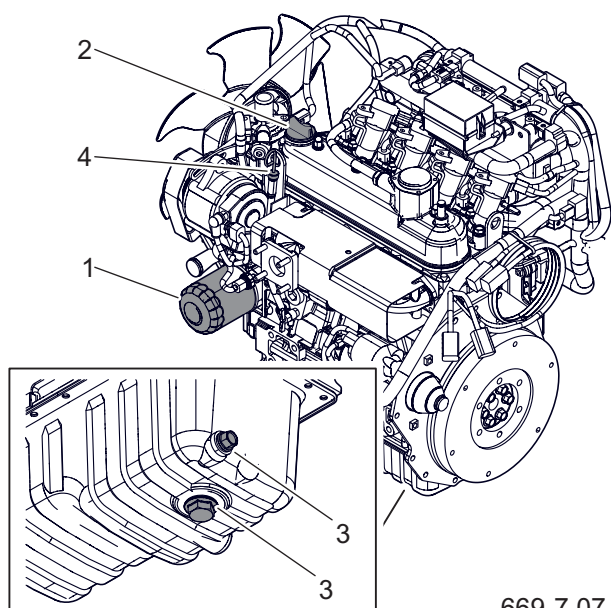
Rysunek 7.9 Olej smarny silnika.
