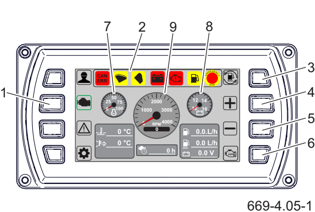
Rysunek 4.5 Ekran silnika (1) przycisk ekran silnika (2) alarmy / ostrzeżenia (3) reset spalania średniego (4) zwiększ obroty (5) zmniejsz obroty (6) bieg jałowy (7) obciążenie silnika (8) napięcie akumulatora (9) obroty silnika
