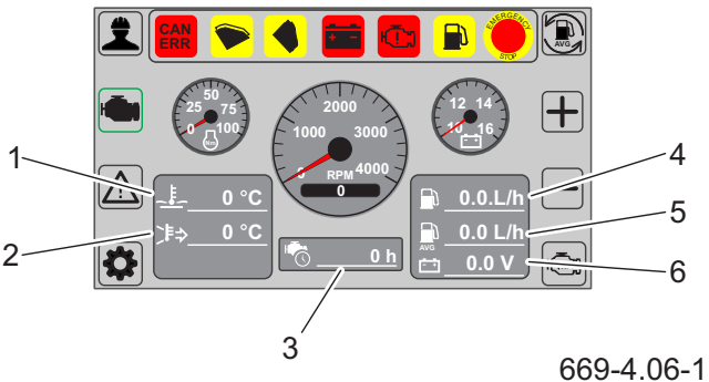
Rysunek 4.6 Ekran silnika (1) temperatura silnika (2) temperatura dolotu silnika (3) czas pracy silnika (4) spalanie chwilowe (5) spalanie średnie (6) napięcie akumulatora
