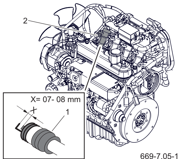
Rysunek 7.7 Świece zapłonowe silnika.
