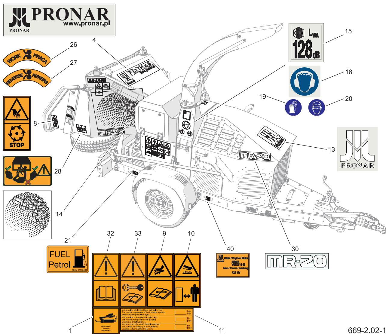
Rysunek 2.2 Rozmieszczenie naklejek informacyjnych i ostrzegawczych.
