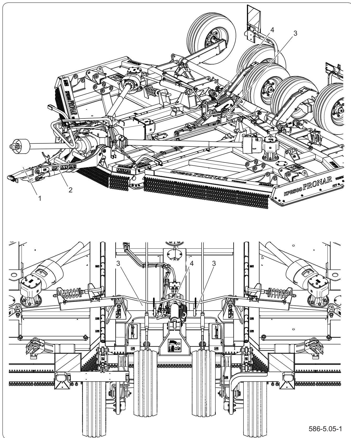
Figure 5.5 Réglage du positionnement de la machine
