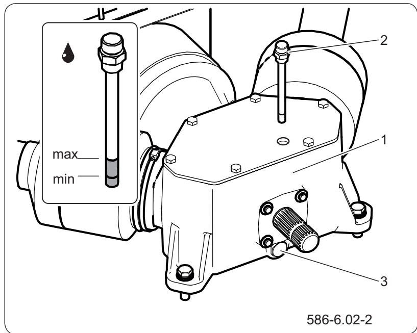
Figure 6.9 Contrôle du niveau et vidange d'huile dans la transmission de distribution
