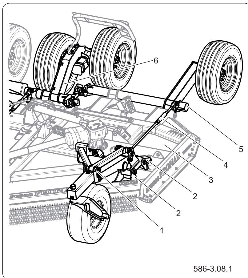
Figure 4.7 Roues copieuses avant
