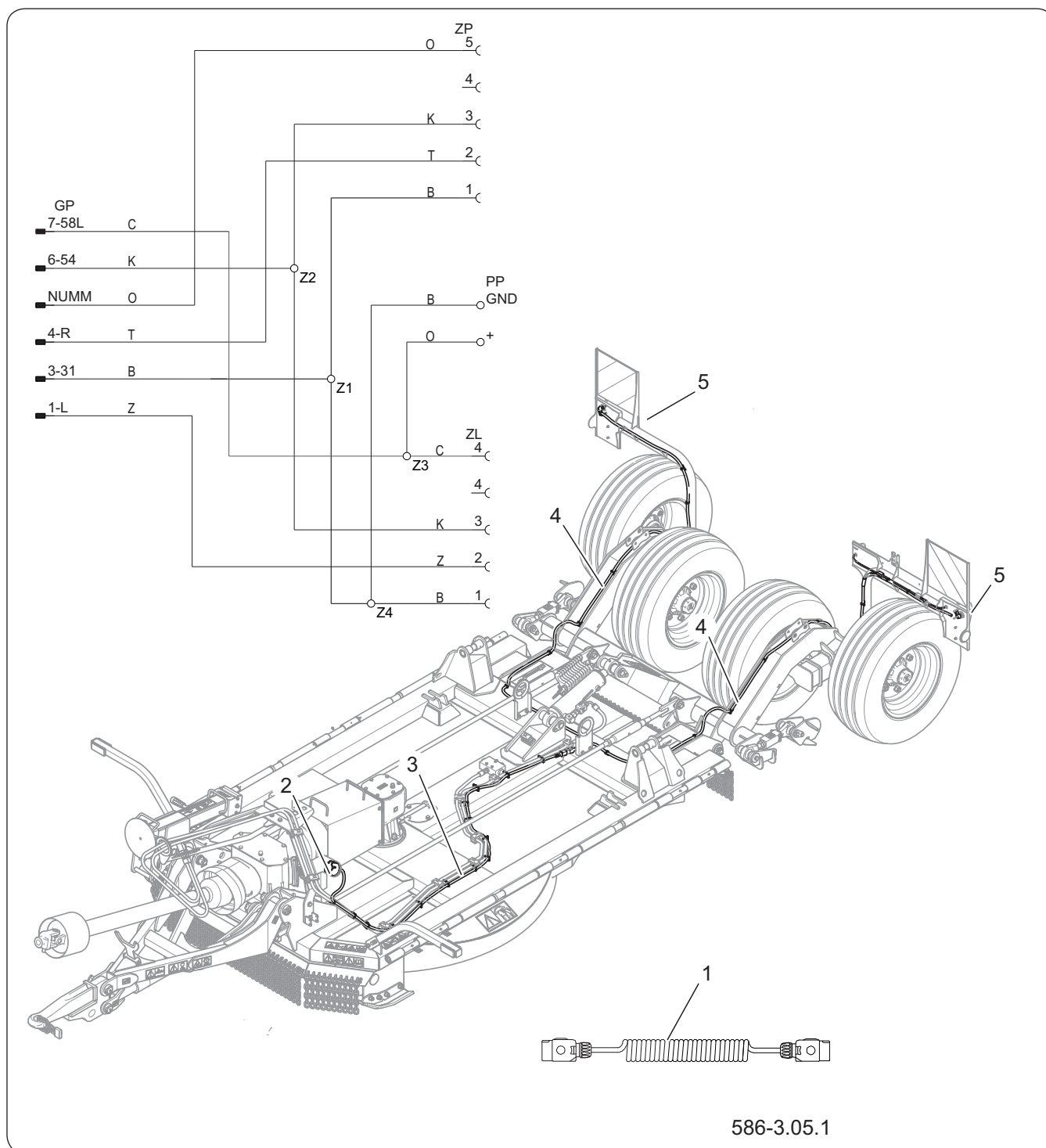
Figure 4.4 Conception de l'installation électrique de la faucheuse KPR500
