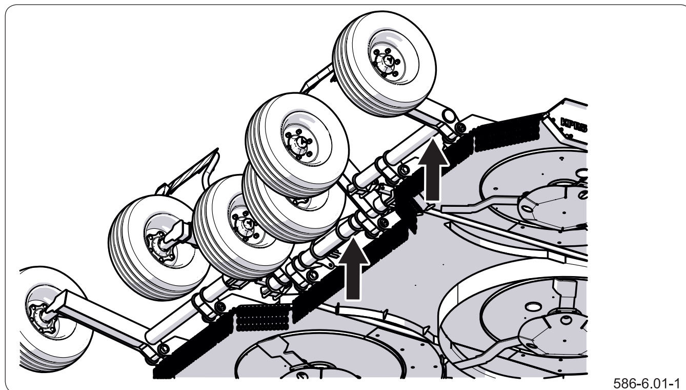
Figure 6.5 Point d'appui du support
