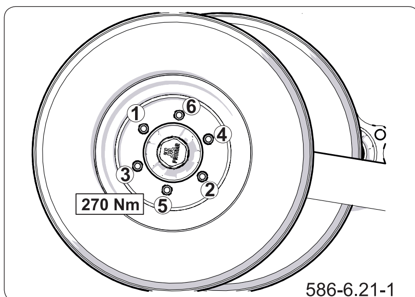
Figure 6.4 Ordre de serrage des écrous
