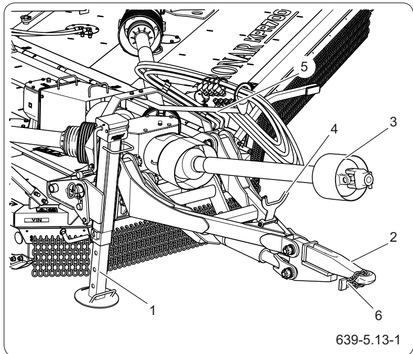
Figure 5.8 Attelage de la faucheuse au porteur
