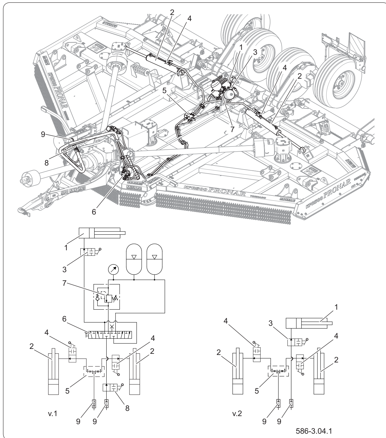
Figure 4.3 Conception du système hydraulique de la faucheuse KPR500 v.1 - version d'installation avec amortissement, v.2 - version d'installation standard (1) cylindre de suspension (2) cylindre d'aile. (3) soupape de cylindre de suspension (4) soupape de cylindre d'aile (5) diviseur de débit (6) distributeur à six voies (7) ensemble d'accumulateur hydraulique (8) soupape d'arrêt (9) fiches de connecteurs hydrauliques
