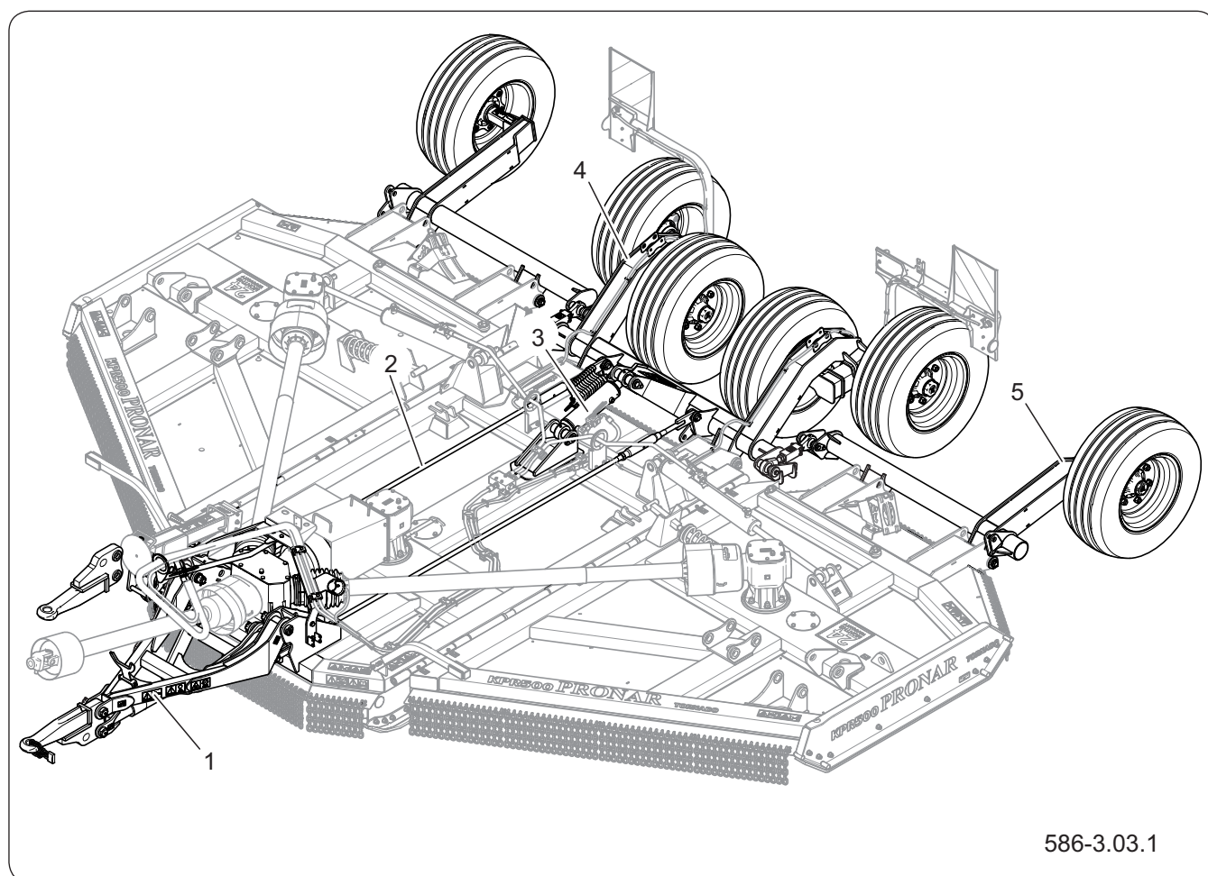
Figure 4.2 Conception du train de roulement
