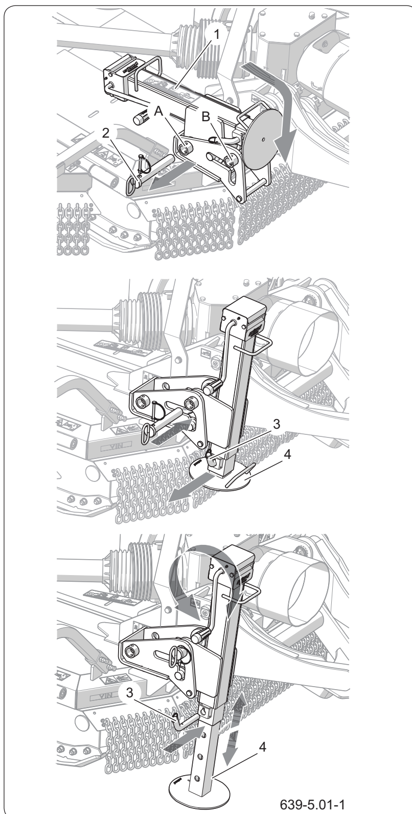
Figure 5.4 Béquille mécanique
