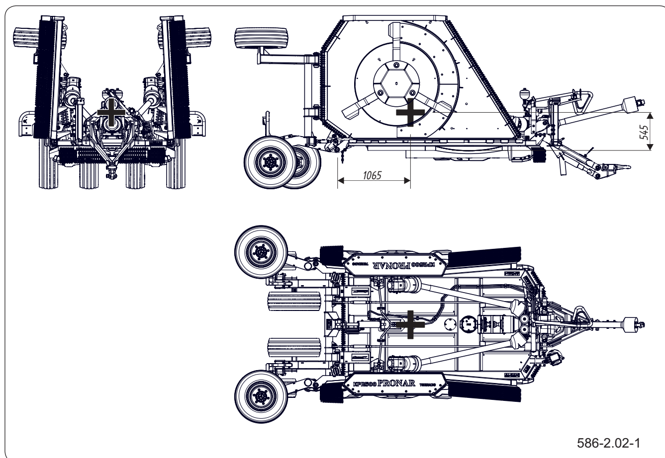
Figure 2.5 Position du centre de gravité de la machine
