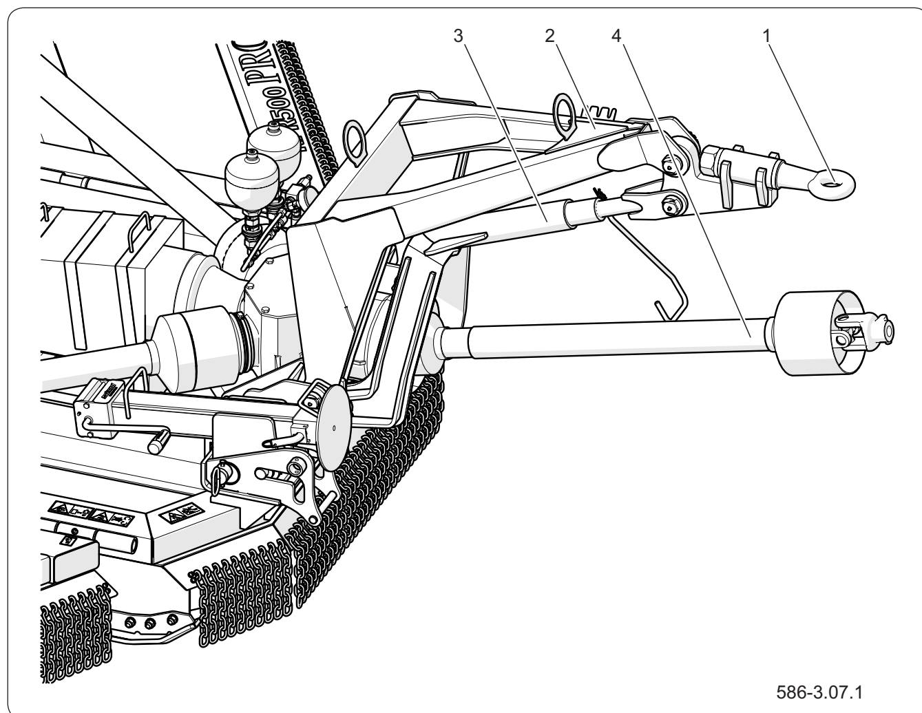
Figure 4.6 Attelage supérieur
