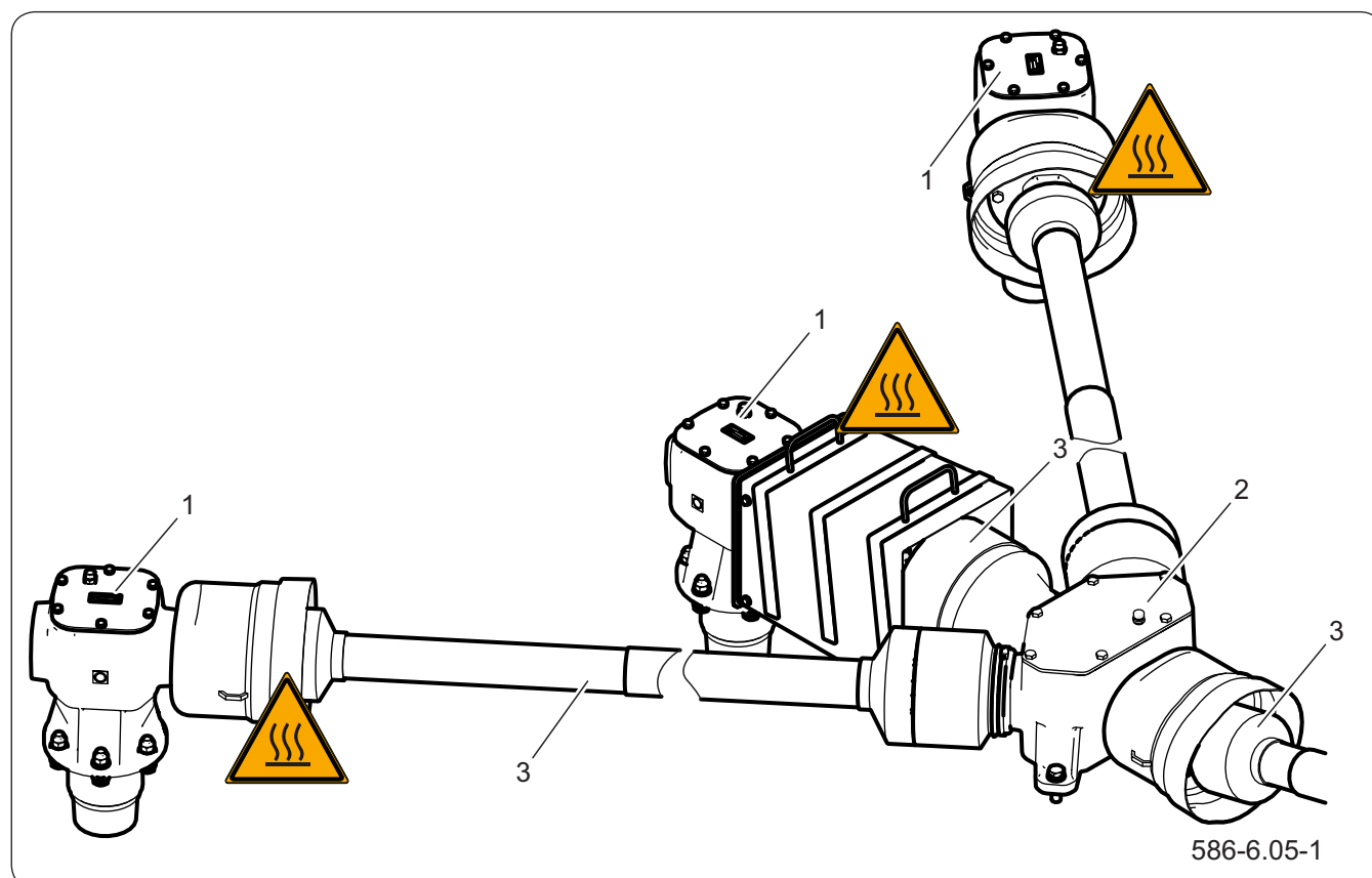
Figure 6.8 Contrôle et vidange d'huile dans la transmission
