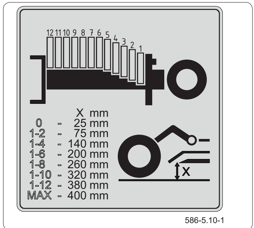
Figure 5.12 Hauteur de fauchage
