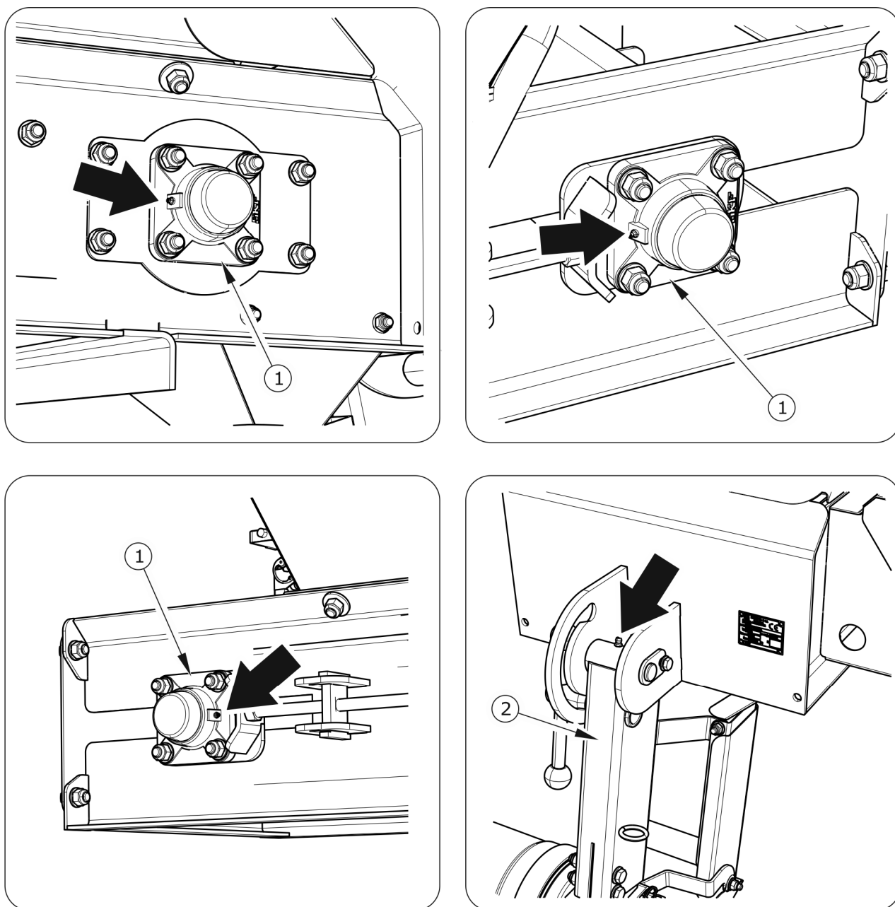
FIGUR 5.1 Smørepunkter på sprederen
