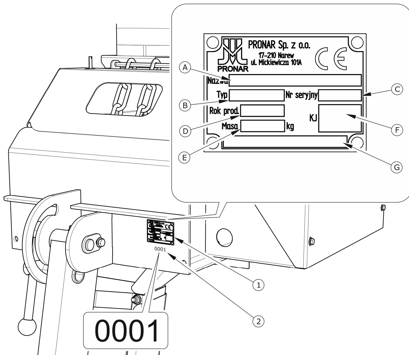
FIGUR 1.1 Placering af typeskiltet og serienummeret
