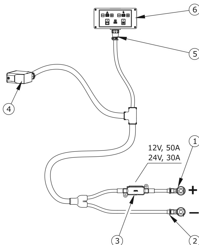
FIGUR 4.4 Tilslutningsledning
