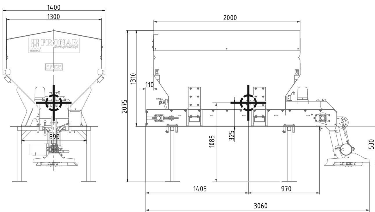
FIGUR 1.4 Tyngdecenter EPT21
