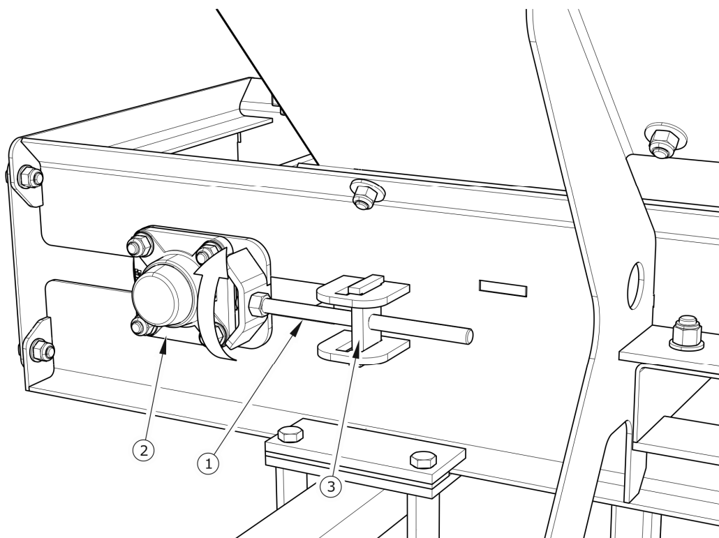
FIGUR 5.3 Justeringsprincip
