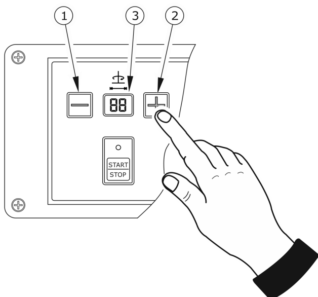
FIGUR 4.6 Breddejustering
