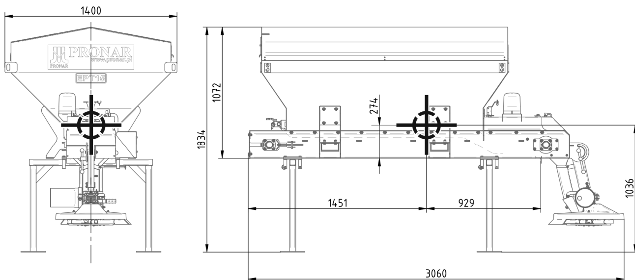
FIGUR 1.3 Tyngdecenter EPT15
