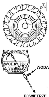
Рисунок 5-27 Способ наполнения колес водой.
