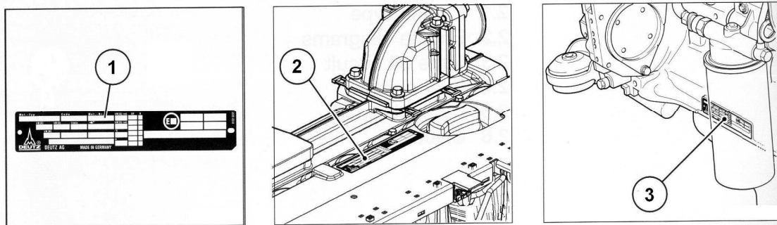
Рисунок 3-2 Расположение заводского щитка 1 двигателя DEUTZ (на крышке 2 и с правой стороны блока-картера двигателя 3)
