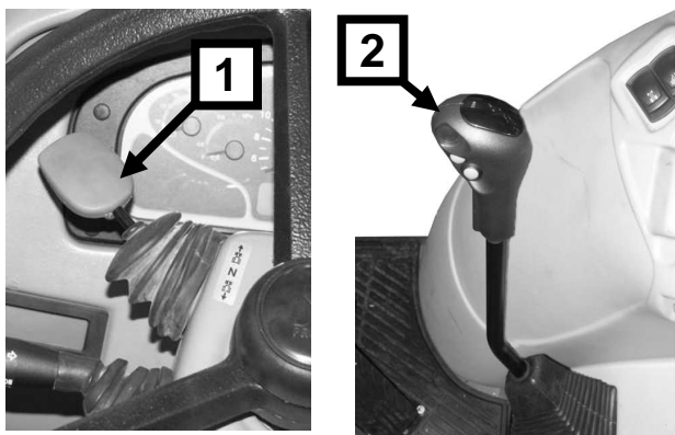
Рисунок 5-5 Рычаг редуктора "черепаха-заяц".
