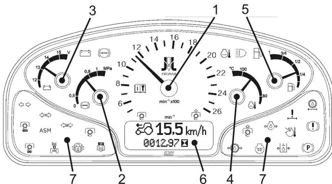
Рисунок 4-10 Контрольно-измерительные приборы в тракторах PRONAR 7150 1 – тахометр; 2 – указатель давления воздуха в пневмосистеме; 3 – указатель напряжения в бортовой сети трактора; 4 – указатель температуры охлаждающей жидкости; 5 – указатель уровня топлива в баке; 6 - счетчик моточасов работы трактора и спидометр; 7 – контрольные лампочки.
