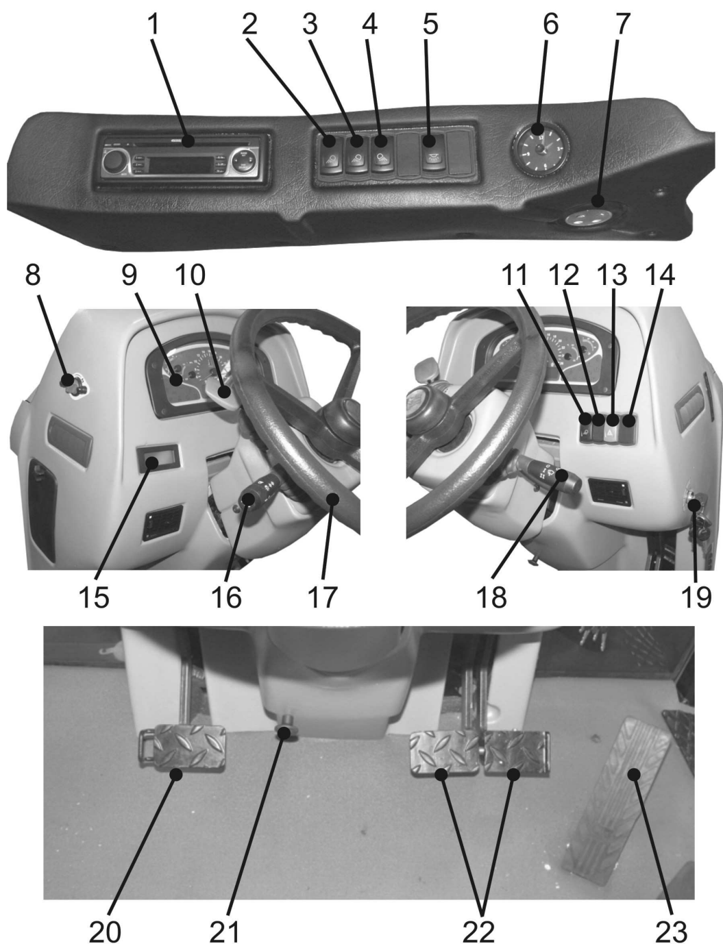
Рисунок 4-7 Расположение органов управления и контрольных приборов в тракторах PRONAR 7150
