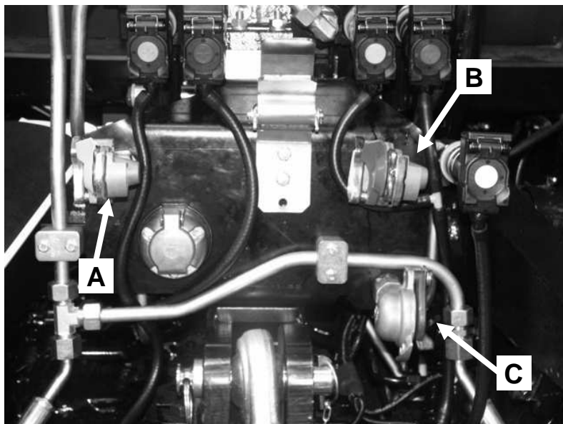
Рисунок 5-24 Соединения пневмосистемы.
