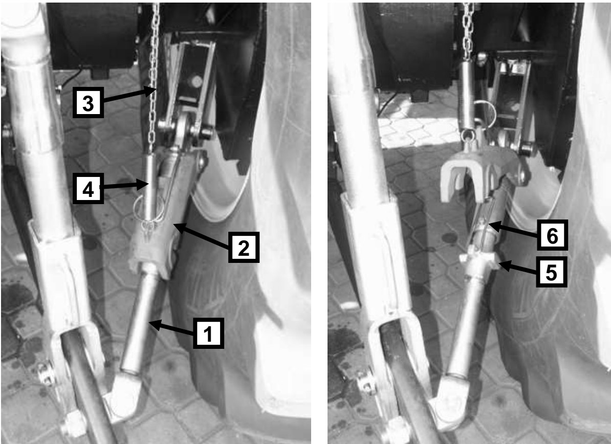
Рисунок 5-13 Стабилизаторы нижних тяг трехточечной системы навески.
