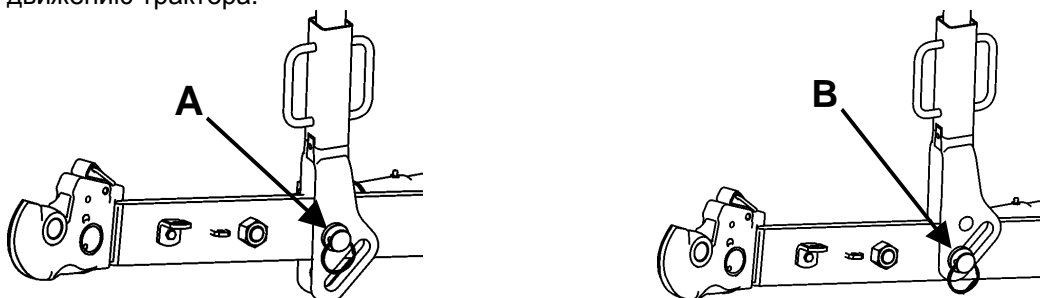
Рисунок 5-11 Способ соединения подвесок с нижними тягово-сцепными устройствами.
