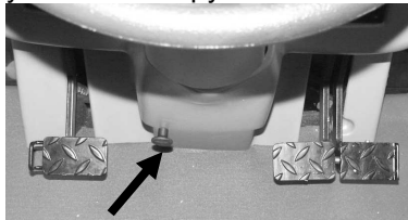
Рисунок 4-22 Ручка блокады угла наклона рулевого колеса (рулевой колонки)
