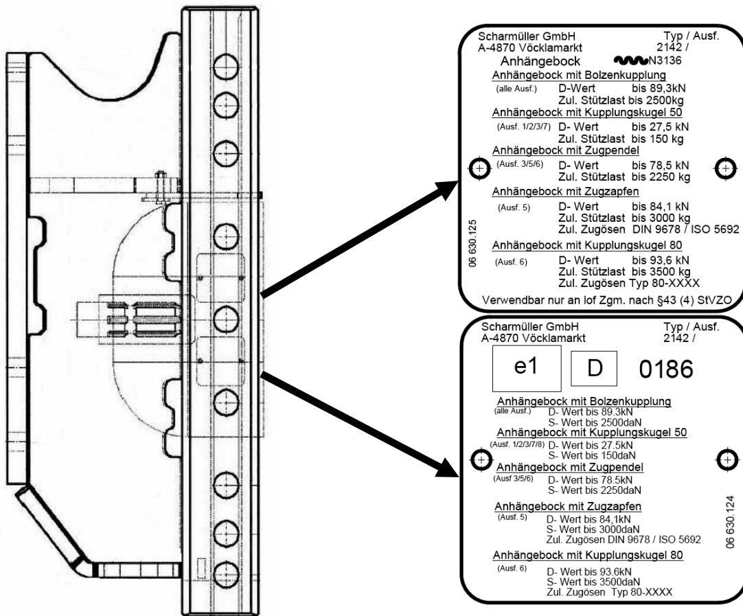
Рисунок 3-5 Расположение заводских щитков монтажных корпусов сцепных устройств
