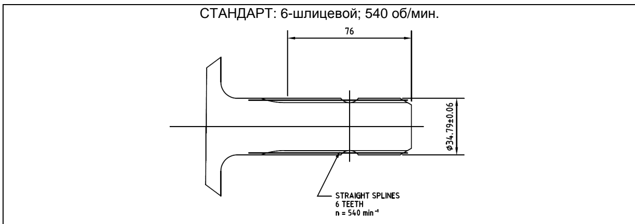
Рисунок 4-29а Размер вала ВОМ в тракторах PRONAR – тип I согл. PN-ISO 500
