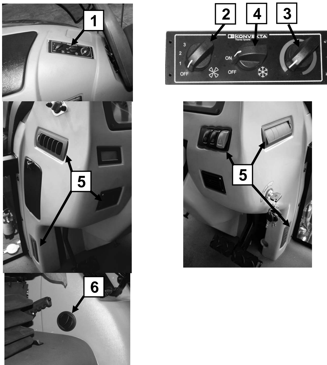
Рисунок 4-21 система отопления, вентиляции и кондиционирования кабины.
