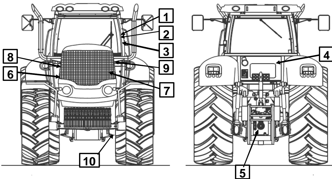
Рисунок 2-1 Расположение предупреждающих знаков на тракторах PRONAR.
