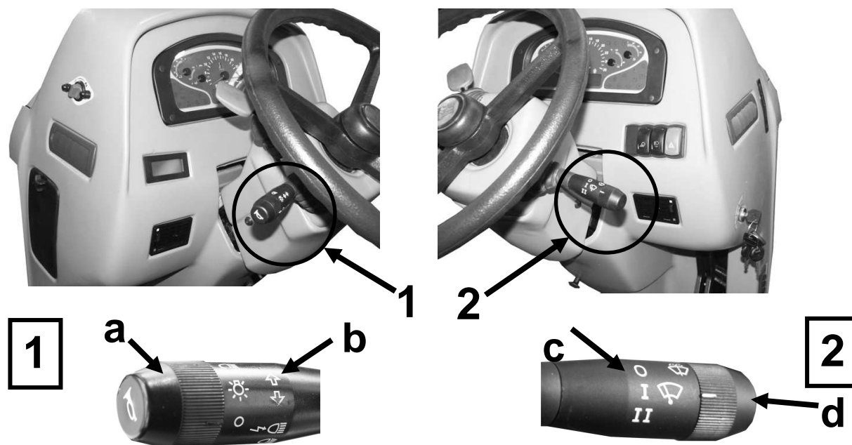
Рисунок 4-13 Многофункциональные переключатели на рулевой колонке: 1 – многофункциональный переключатель света и звукового сигнала 2 - многофункциональный включатель стеклоочистителей и омывателя лобового стекла
