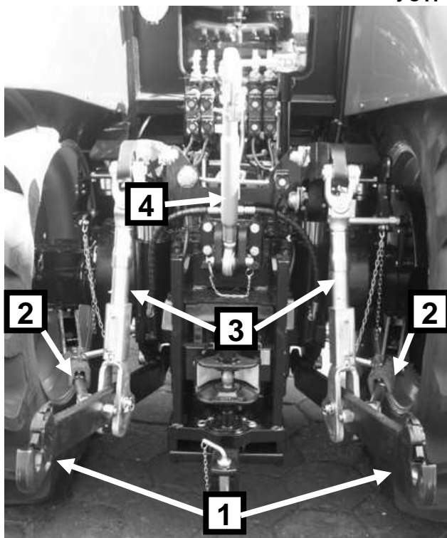
Рисунок 5-8 Трехточечная система навески – устройство.
