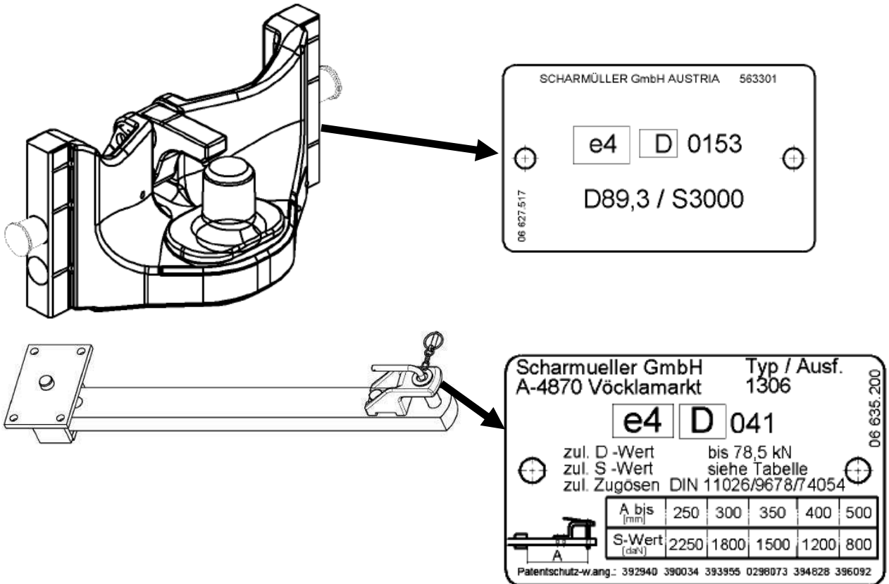
Рисунок 3-6 Расположение заводских щитков сцепных устройств
