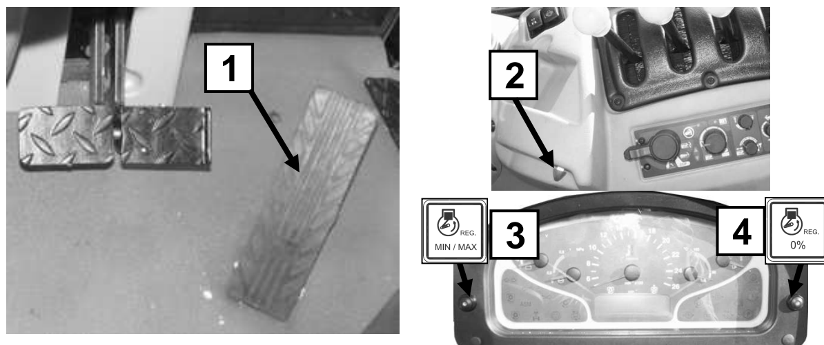
Рисунок 4-15 Управление скоростью вращения двигателя. 1 – педаль управления подачей топлива; 2 – рычаг управления подачей топлива; 3 – кнопка режима работы регулятора числа оборотов двигателя; 4 – кнопка выбора жесткости работы регулятора числа оборотов двигателя.
