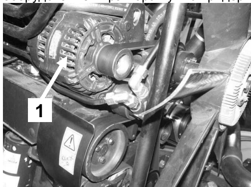
Рисунок 5-28 Альтернатор
