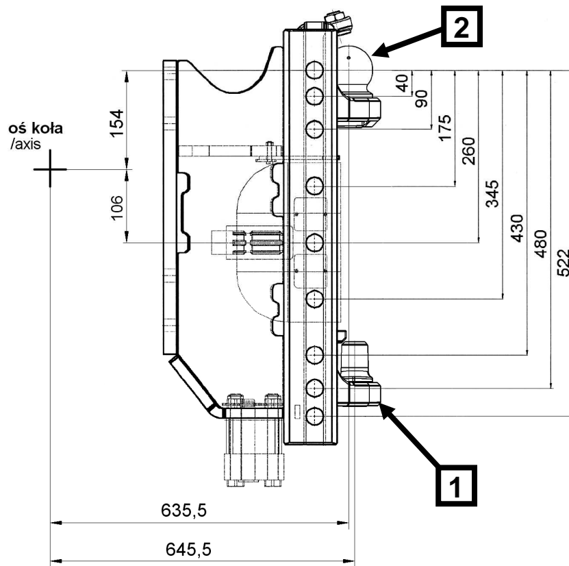
Рисунок 5-17 Сцепка для одноосных прицепов тип PİTONFIX (1) и шаровая сцепка Ø80 (2) - габариты
