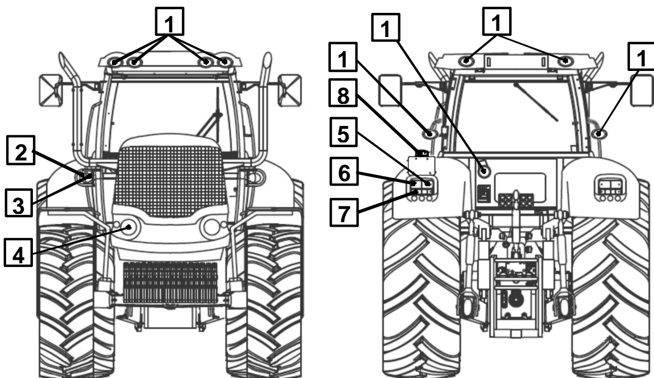
Рисунок 5-35 Система световой сигнализации трактора.
