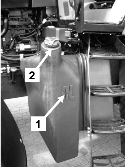
Рисунок 5-36 Топливный бак. 1 – топливный бак с левой стороны трактора; 2 – заливная пробка топливного бака
