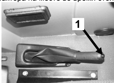
Рисунок 4-25 Стояночный тормоз. 1- кнопка на рычаге стояночного тормоза
