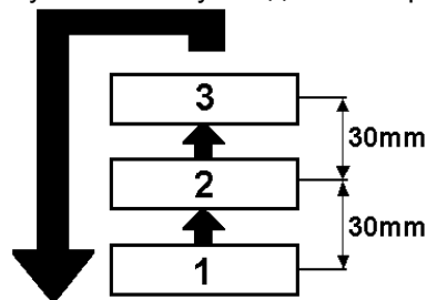
Рисунок 4-17 Три положения сиденья GRAMMER по высоте.
