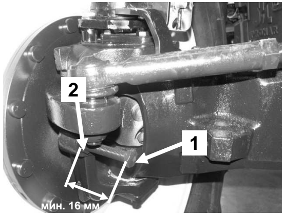
Рисунок 5-25 Регулирование угла поворота передних колес.
