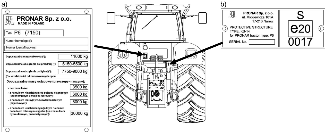
Рисунок 3-1 Расположение заводских щитков.
