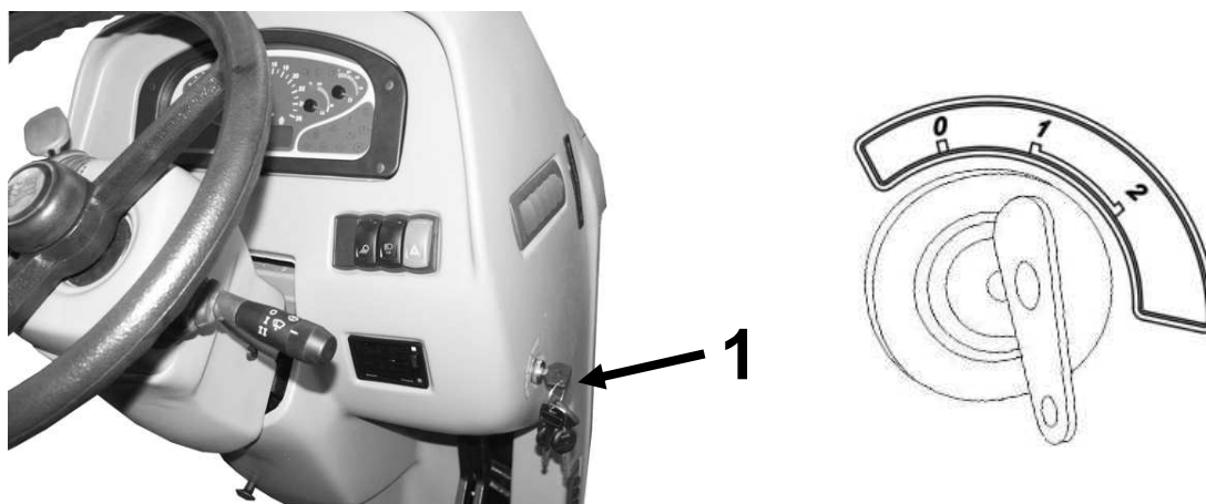
Рисунок 4-14 Управление пуском двигателя: 1 – замок зажигания;
