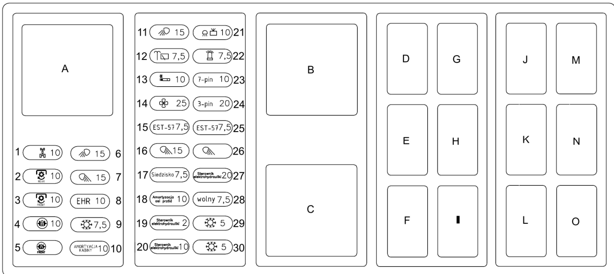
Рисунок 5-34 Обозначения предохранителей в коробке предохранителей на рулевой колонке (FB1 и FB2) и на крыле с правой стороны сиденья (FB3 и FB4).
