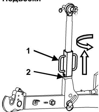
Рисунок 5-10 Трехточечная система навески. 1- стяжной болт с рукояткой; 2- блокировка.
