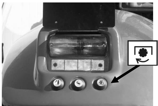
Рисунок 4-31 Выключатель ВОМ на левом заднем крыле трактора.
