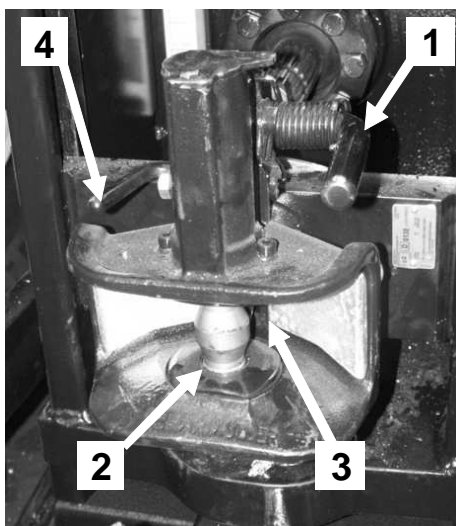
Рисунок 5-15 Верхнее буксирное устройство автоматического типа.
