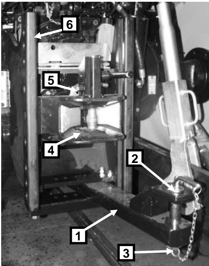
Рисунок 5-14 Тягово-сцепные устройства в тракторах PRONAR – устройство. 1 – сельскохозяйственная сцепка; 2 – шкворень сельскохозяйственной сцепки; 3 – шплинт шкворня сельскохозяйственной сцепки; 4 – буксирное устройство; 5 – рычаг регулирования буксирного устройства в вертикальной плоскости; 6 – направляющие для регулирования буксирного устройства в вертикальной плоскости;
