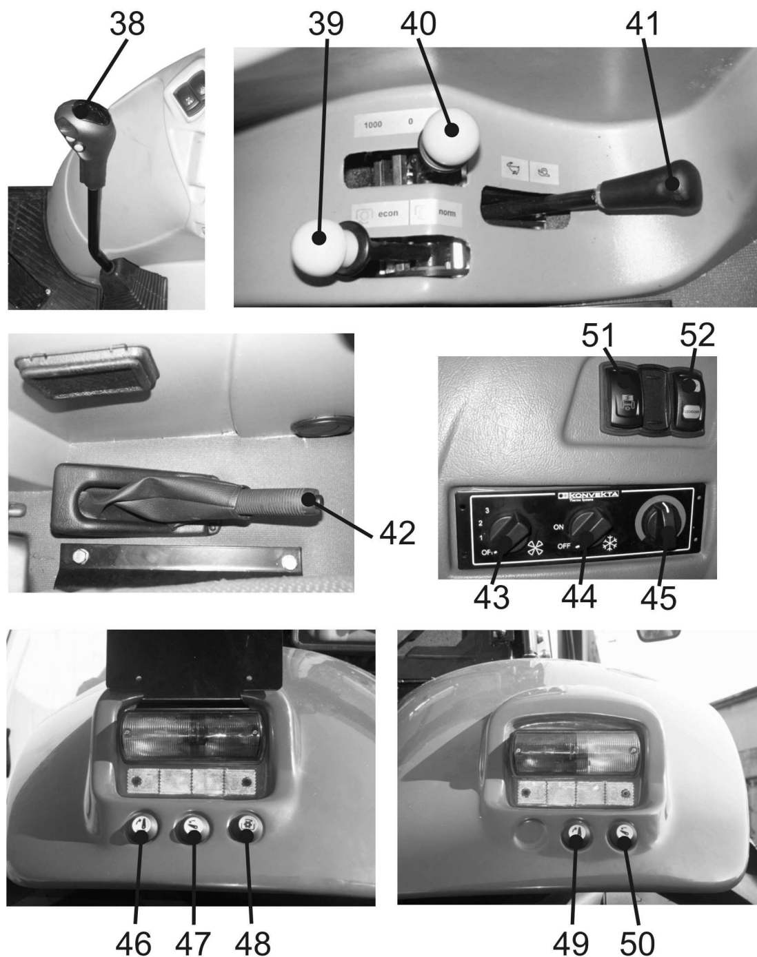
Рисунок 4-9 Расположение органов управления и контрольных приборов в тракторах PRONAR 7150.
