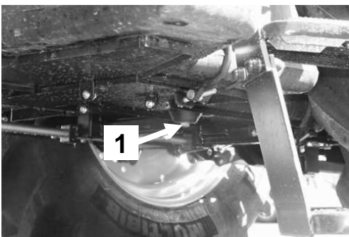
Рисунок 5-37 Сливная пробка топливного бака. 1 – сливная пробка топливного бака. После слива топлива или удаления осадка нужно завинтить пробку.
