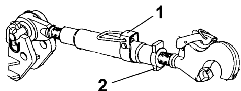
Рисунок 5-12 Регулирование верхнего тягово-сцепного устройства трехточечной системы навески.
