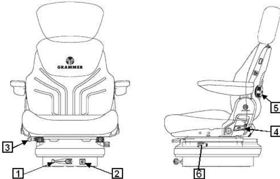
Рисунок 4-16 Расположение регулирующих механизмов сиденья GRAMMER MSG85/721 и DS 85H/90A
