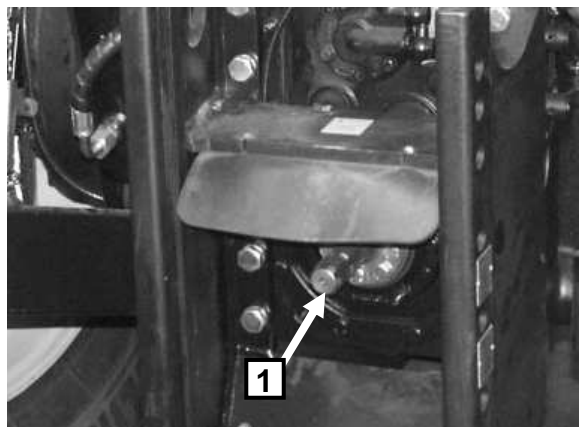
Рисунок 4-32 Конец вала ВОМ.
