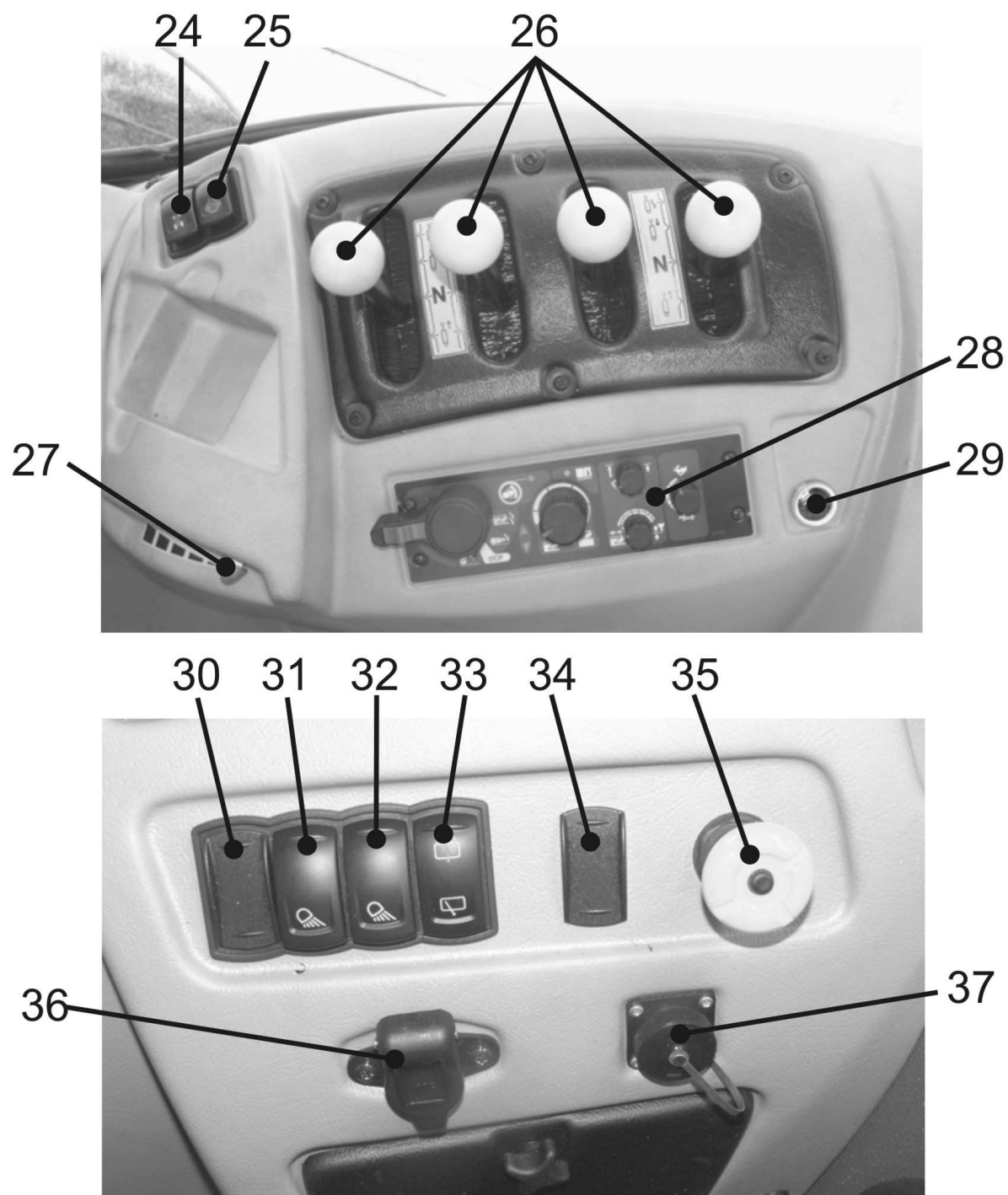
Рисунок 4-8 Расположение органов управления и контрольных приборов в тракторах PRONAR 7150.
