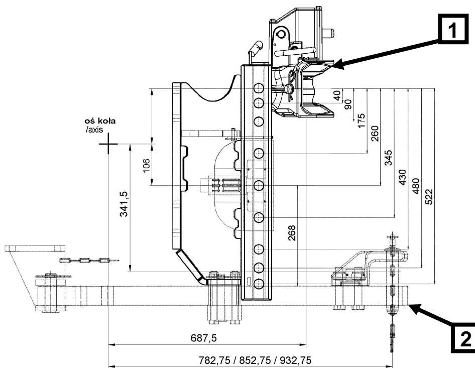
Рисунок 5-16 Автоматическое буксирное устройство (1) и сельскохозяйственная сцепка (2) - габариты
