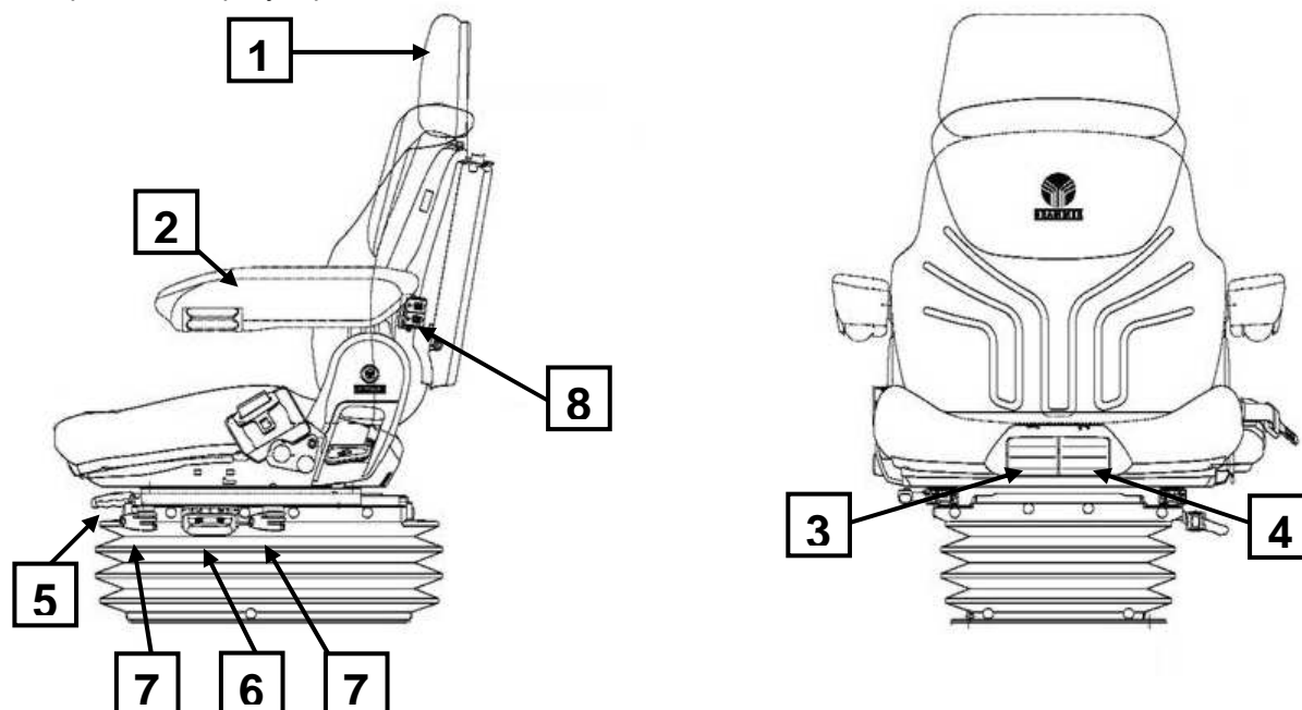
Рисунок 4-18 Расположение регулирующих механизмов сиденья GRAMMER MSG 95 AL./731 1- регулируемый подголовник; 2- подлокотник; 3- клавиш перемещения сиденья вперед или назад; 4- клавиш положения сиденья по высоте; 5- рычаг продольного регулирования подвески сиденья; 6- клавиш регулирования пневматической подвески сиденья; 7- ограничители, гасящие вибрации сиденья; 8- клавиш регулирования опоры для поясницы;
