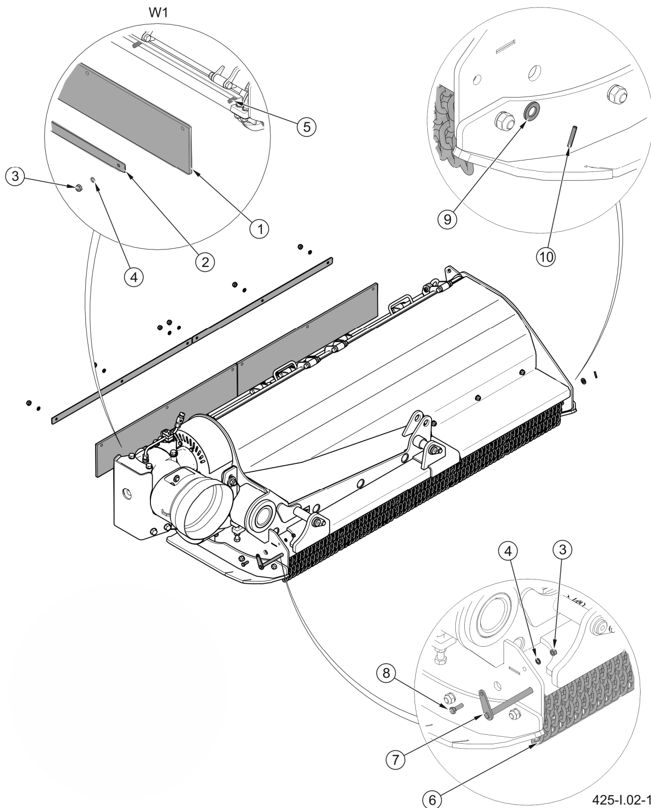
RYСУNEK 5.2 Demontaż osłony
