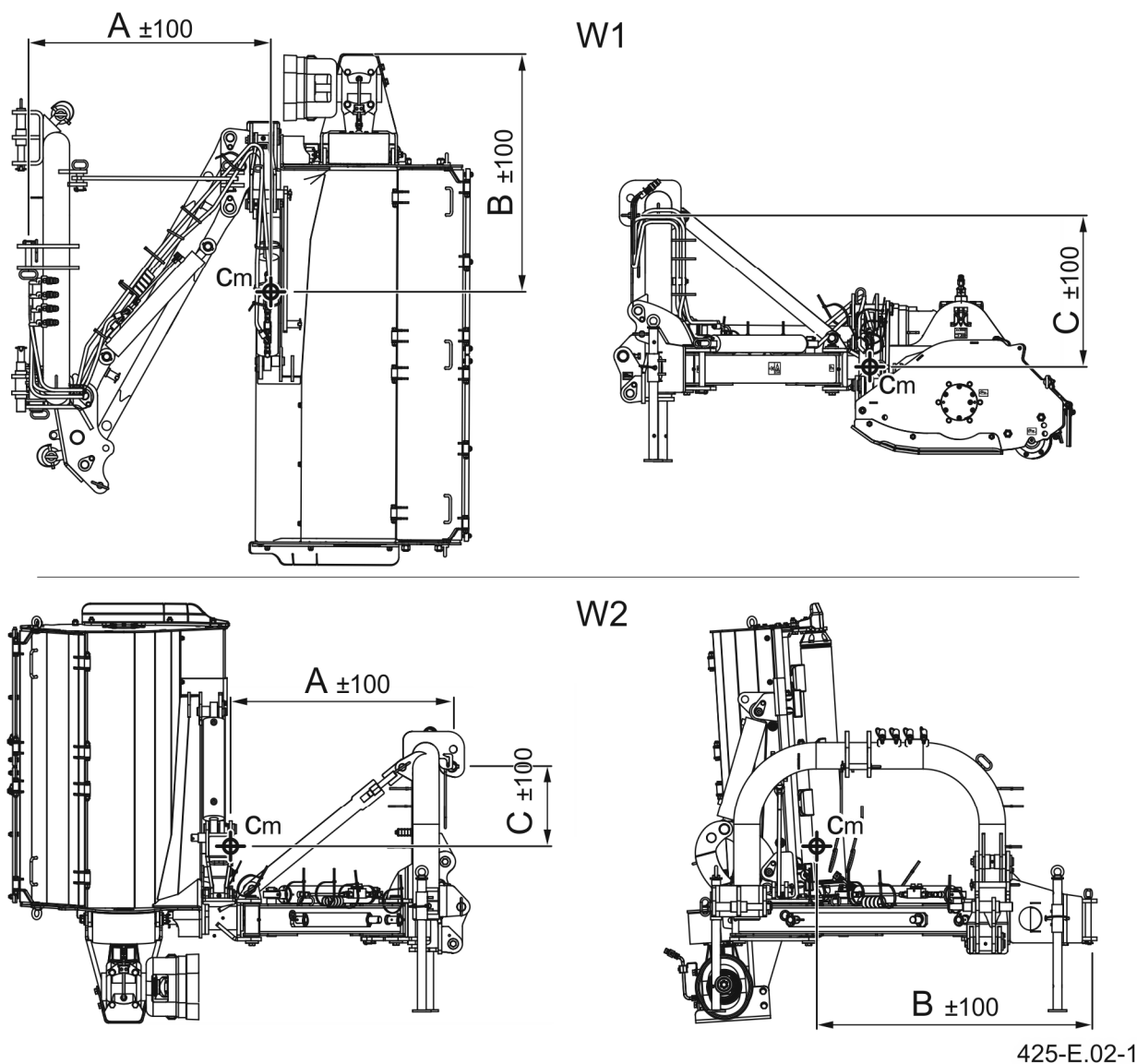
RYSUNEK 1.2 Położenie środka ciężkości kosiarki
