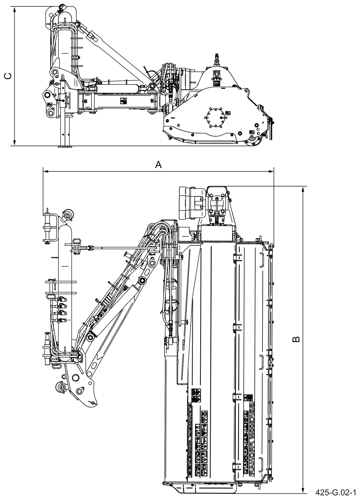
RYSUNEK 3.2 Wymiary gabarytowe kosiarki
