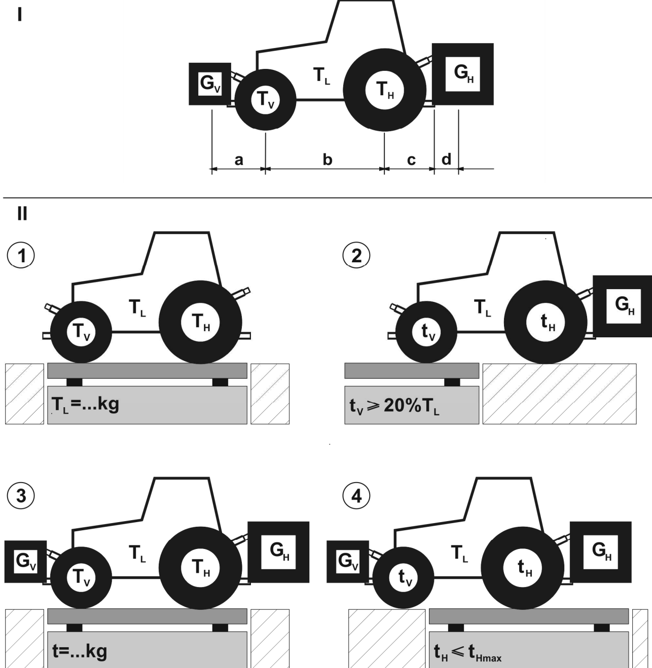
RYSUNEK 4.2 Dociążenie ciągnika
