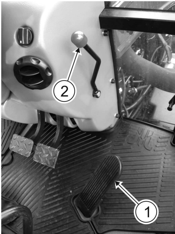
RYСУNEK 3.15 Sterowanie prędkością obrotową silnika.
