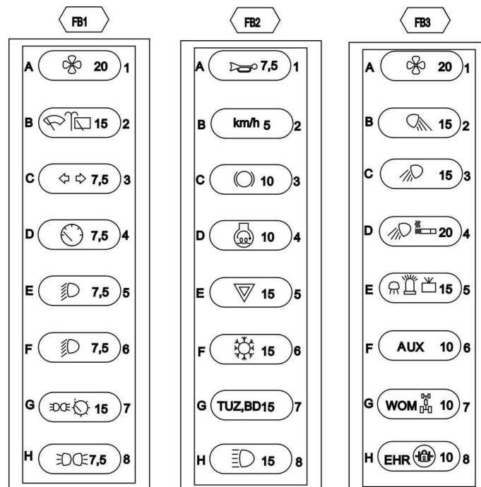
RYSUNEK 4.44 Opis zestawów bezpieczników ciągników PRONAR
