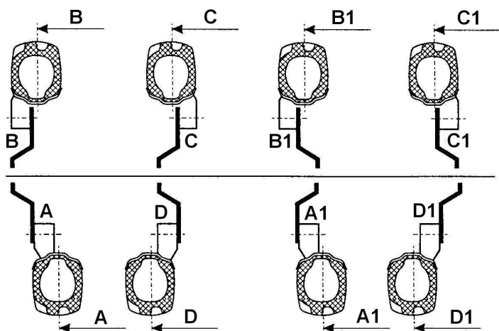
RYСУNEK 4.34 Schemat rozstawu kół przedniego mostu napędowego
