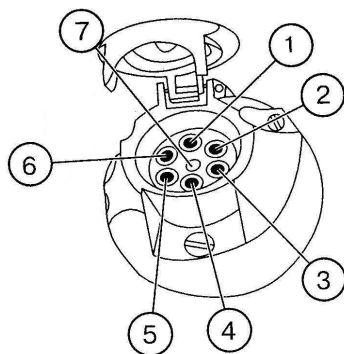
RYSUNEK 4.40 Złącze instalacji elektrycznej dla przyczep
