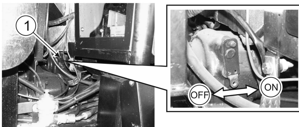
RYSUNEK 4.26 Dźwignia włączania pompy układu hydraulicznego
