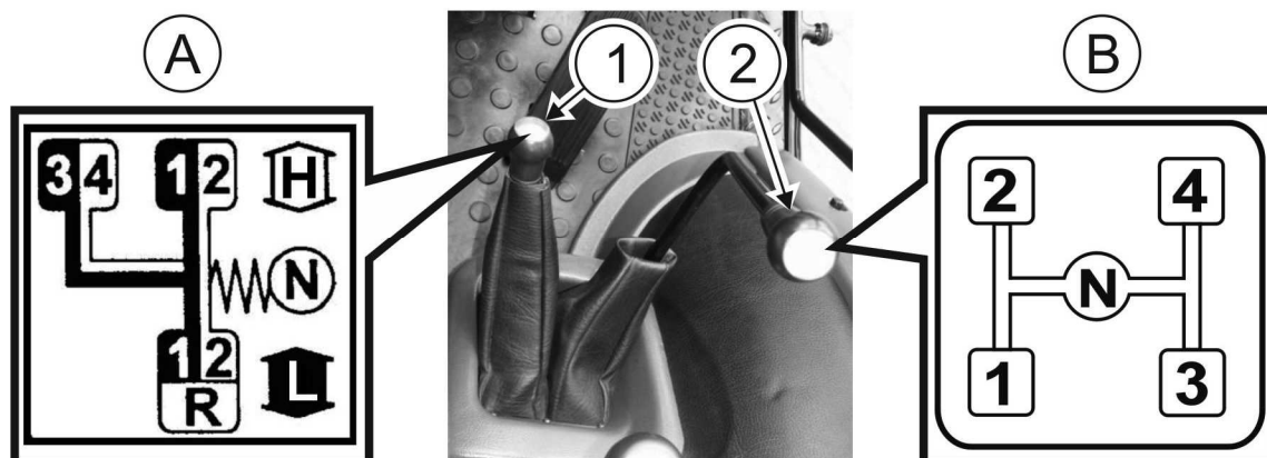
RYSUNEK 4.8 Dźwignie zmiany biegów
