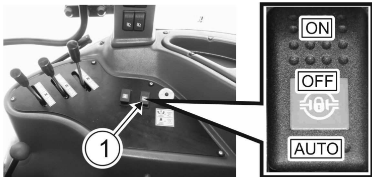
RYSUNEK 3.28 Sterowanie blokadą mechanizmu różnicowego tylnego mostu
