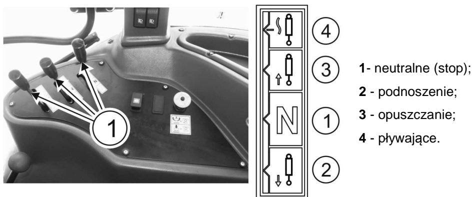
RYSUNEK 4.27 Dźwignie i piktogram sterowania układem hydrauliki zewnętrznej
