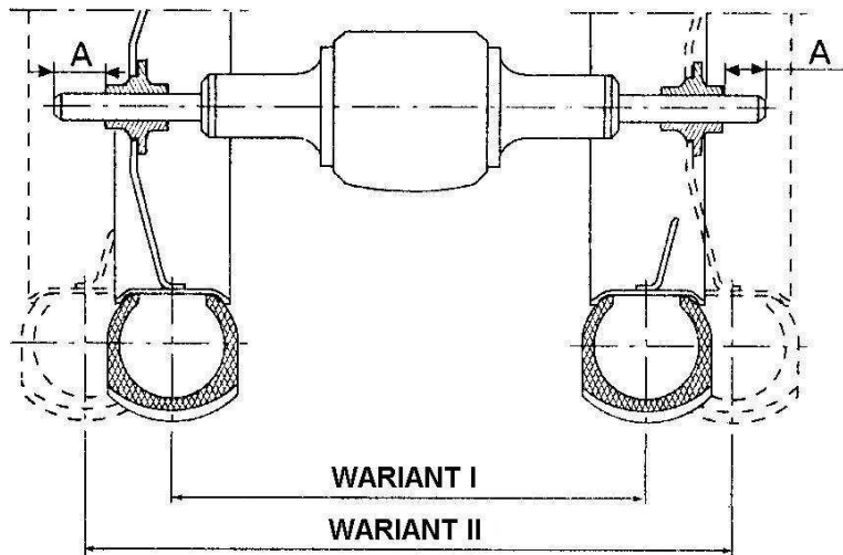
RYSUNEK 4.35 Schemat ideowy zmiany rozstawu kół tylnych
