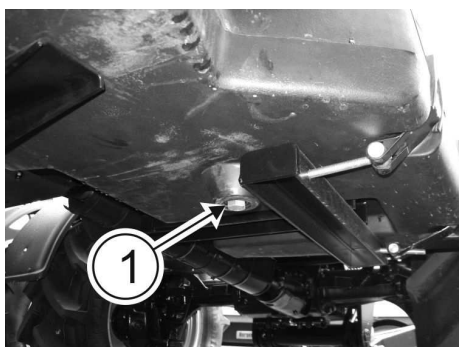
RYSUNEK 4.46 Korek spustowy zbiornika paliwa
