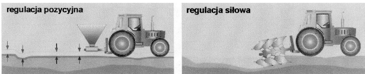
RYSUNEK 4.23 Sposoby regulacji stosowanej w podnośnikach ciągników rolniczych.
