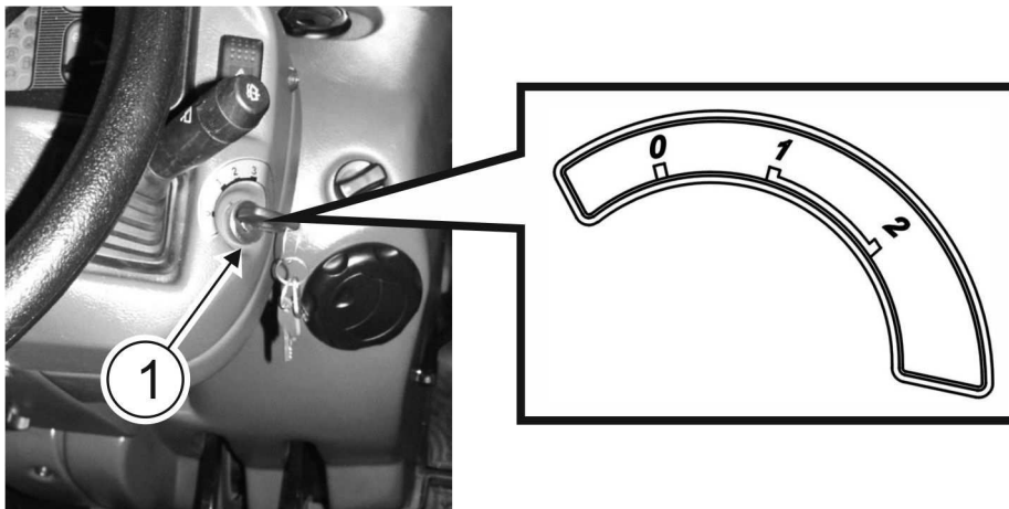
RYSUNEK 3.14 Sterowanie rozruchem silnika.
