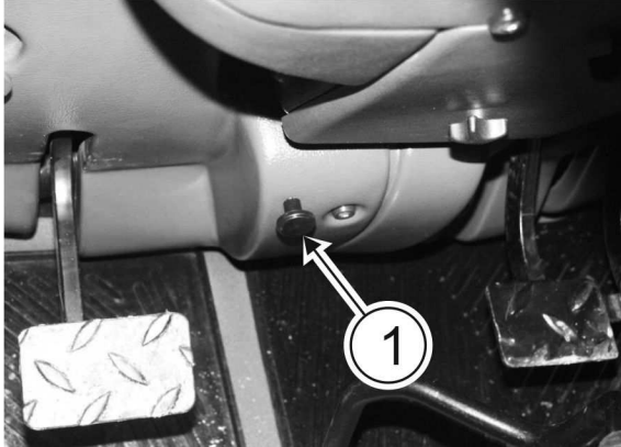
RYSUNEK 3.23 Cięgło blokady nachylenia koła (kolumny) kierownicy.
