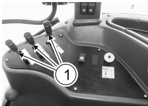
RYSUNEK 4.22 Dźwignie sterujące wyjściami hydrauliki zewnętrznej
