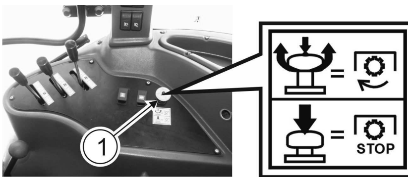
RYSUNEK 3.33 Włączanie WOM-u.
