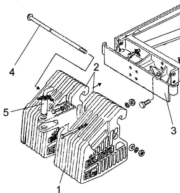
RYSUNEK 4.37 Obciążniki przednie.
