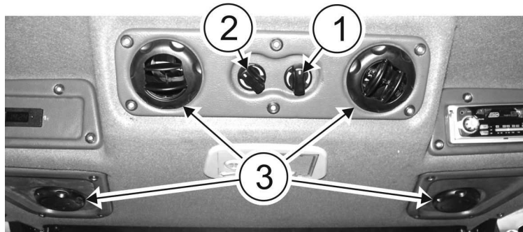
RYSUNEK 3.22 Układ klimatyzatora kabiny (opcja).
