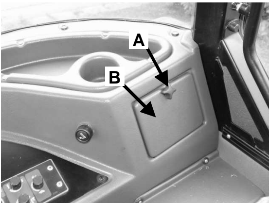
RYSUNEK 4.43 Położenie zestawu bezpieczników FB3 na prawym nadkolu.
