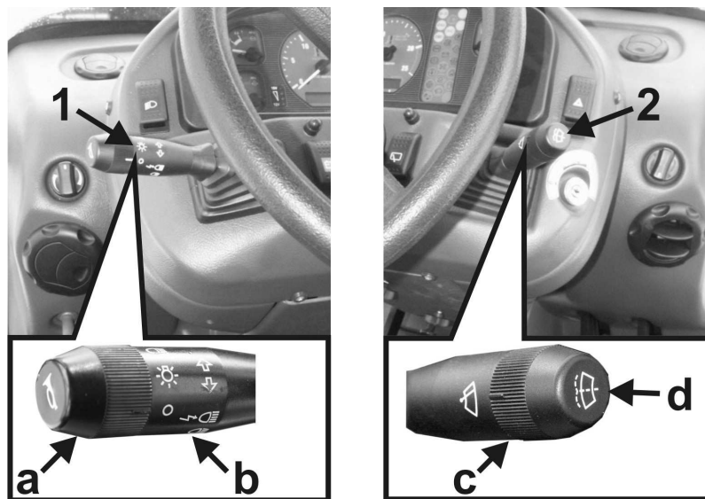
RYSUNEK 3.13 Włączniki wielofunkcyjne przy kolumnie kierowniczej.
