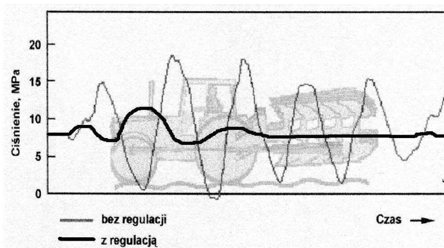
RYSUNEK 4.24 Wykres tłumienia drgań.
