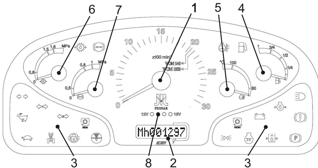
RYСУNEK 3.10 Wskaźniki kontrolne
