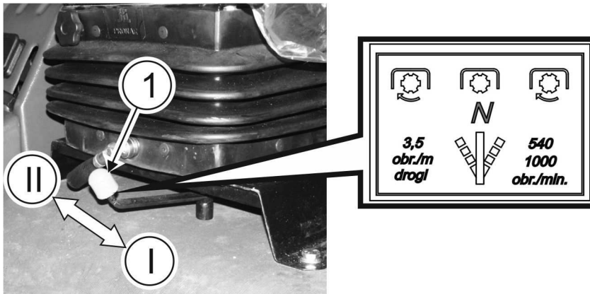
RYSUNEK 3.29 Dźwignia wyboru obrotów ZALEŻNE – NIEZALEŻNE WOM
