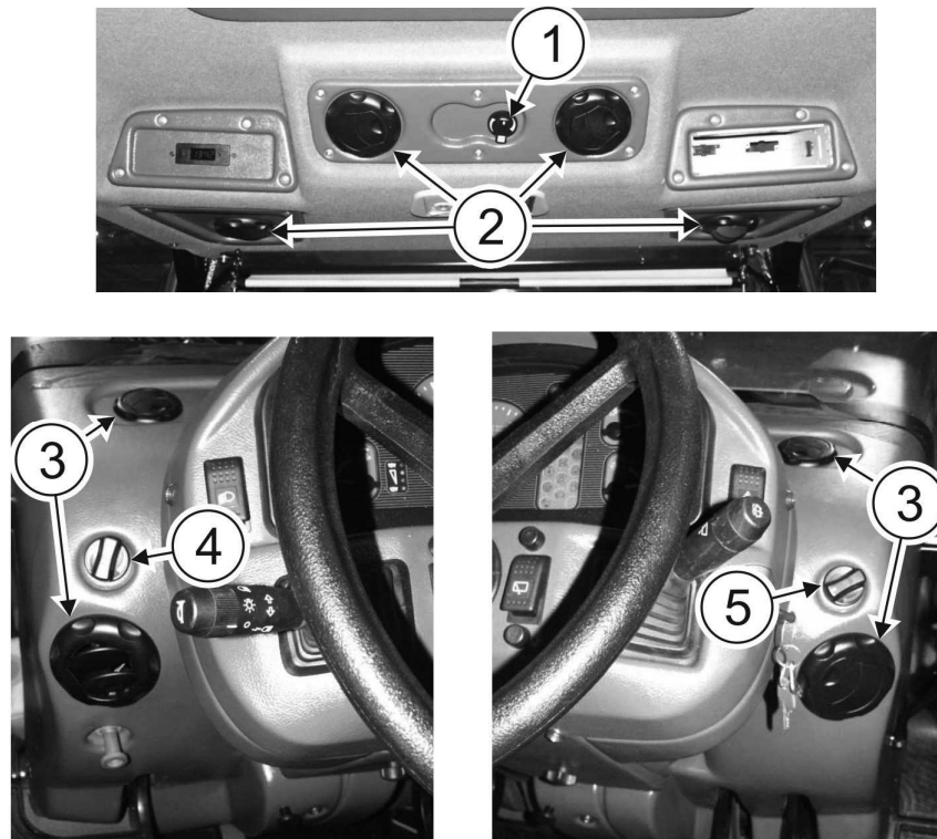
RYСУNEK 3.21 Układ wentylacji i ogrzewania kabiny
