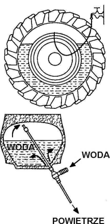
RYSUNEK 4.38 Sposób napełniania kół wodą
