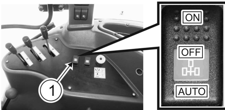
RYSUNEK 3.27 Włącznik sterowania napędem przedniego mostu.
