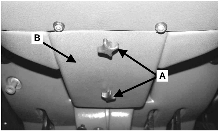
RYSUNEK 4.42 Położenie zestawu bezpieczników FB1 i FB2 przy kolumnie kierowniczej.
