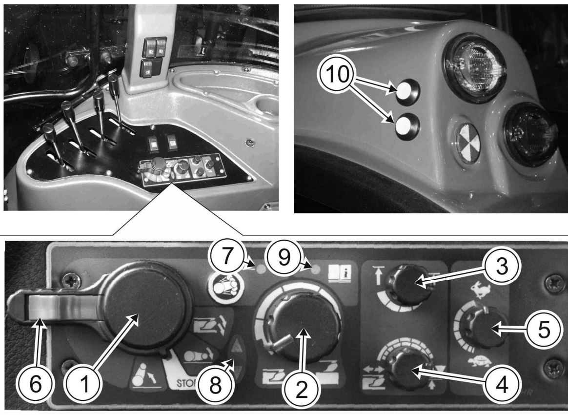
RYSUNEK 4.25 Panel sterowania układem elektrohydraulicznym EHR.
