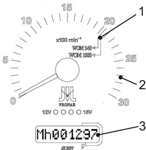
RYСУNEK 3.11 Obrotomierz.
