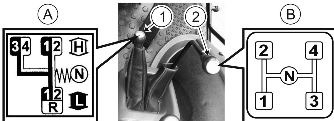
RYSUNEK 4.3 Dźwignie zmiany biegów
