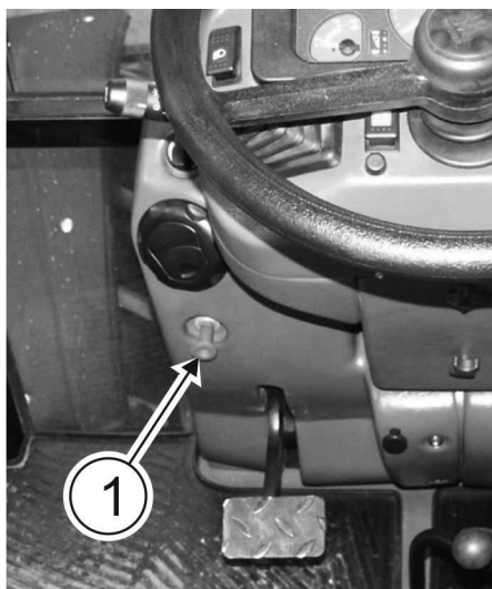
RYSUNEK 4.10 Cięgło zatrzymania silnika
