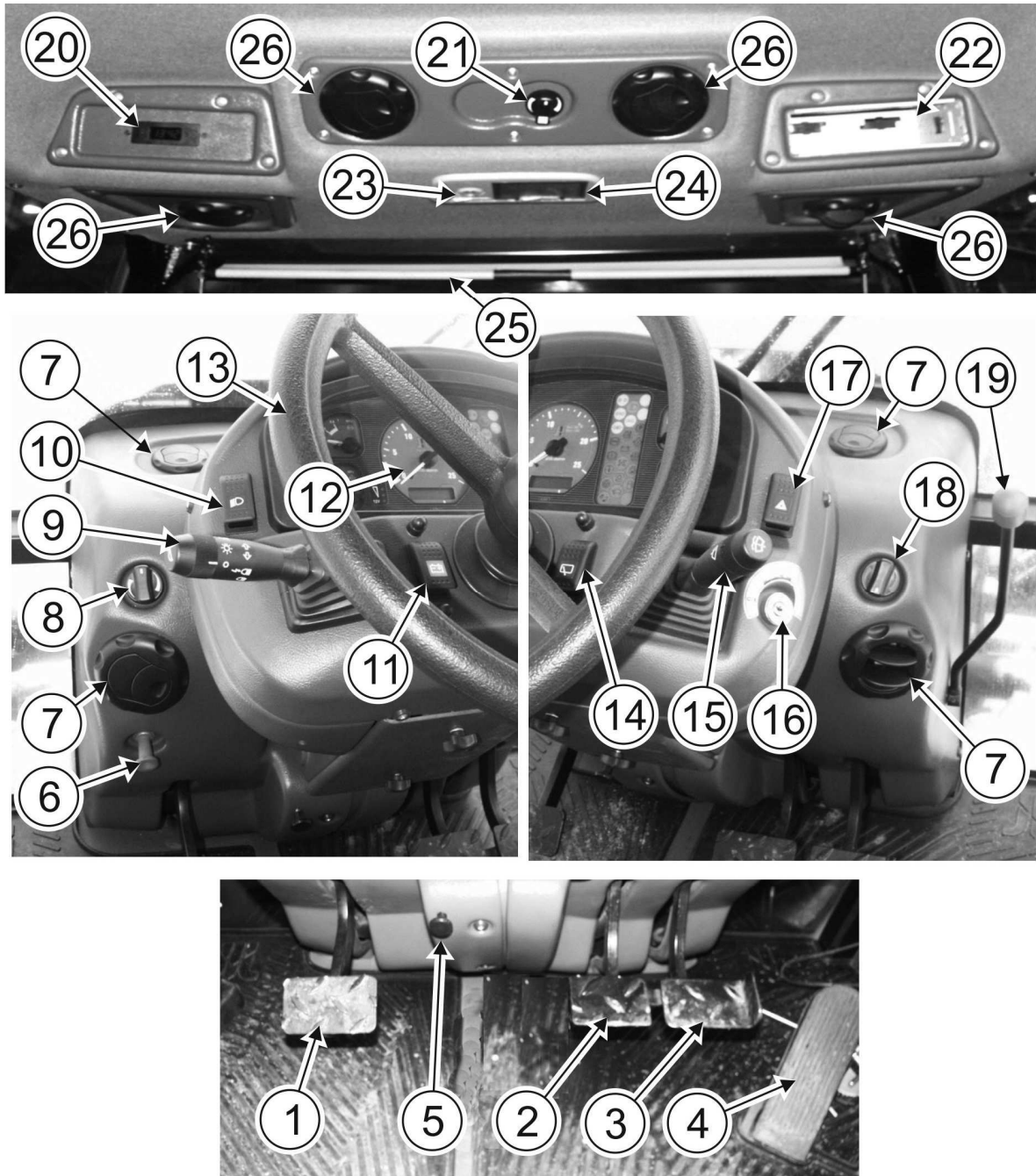
RYSUNEK 3.8 Usytuowanie organów sterowania i kontroli PRONAR 1221A II
