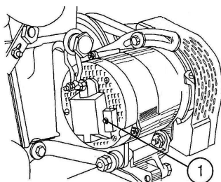
RYSUNEK 4.39 Alternator
