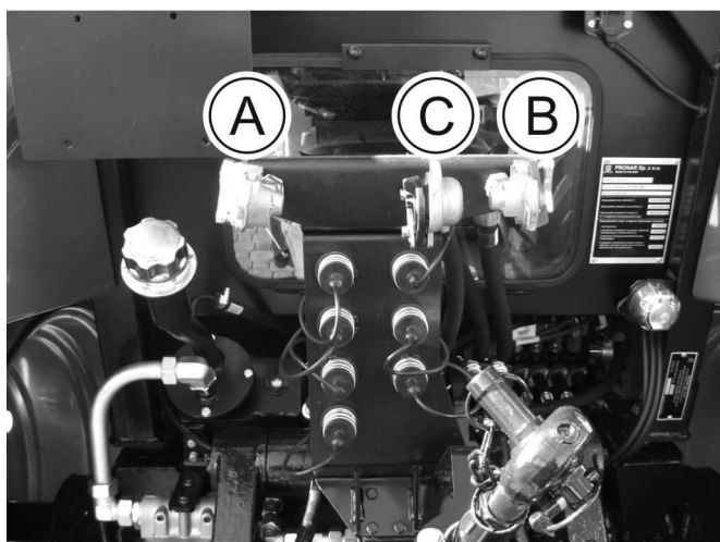
RYSUNEK 4.33 Złącza układu pneumatycznego.
