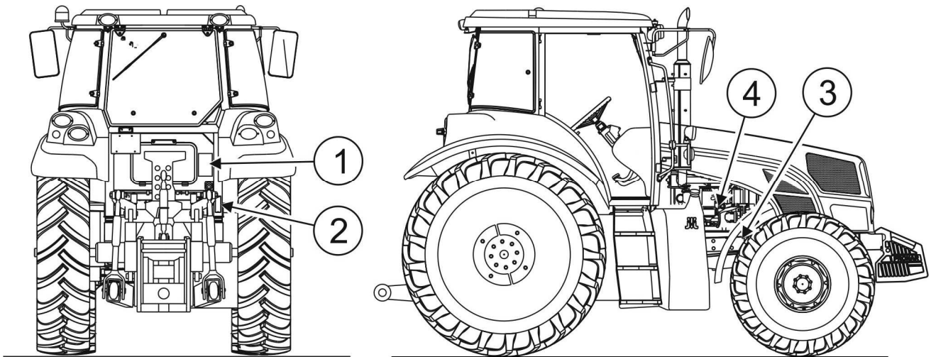
RYSUNEK 1.1 Położenie tabliczek producenta.
