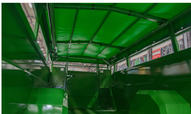
Dimension intérieure du pont : longueur 6290 mm, largeur 2240 mm, hauteur 2100 mm
