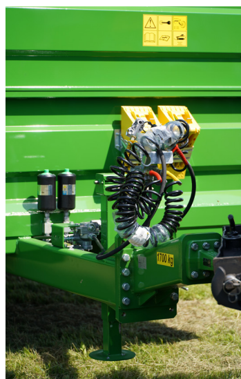
Béquille mécanique avec manivelle fournie dans l'équipement standard
