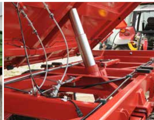
Robustes Fahrgestell durch rechteckige geschlossene Stahlprofile
