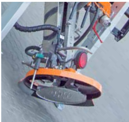
Układ zasypowy z tarczą rozsiewającą
